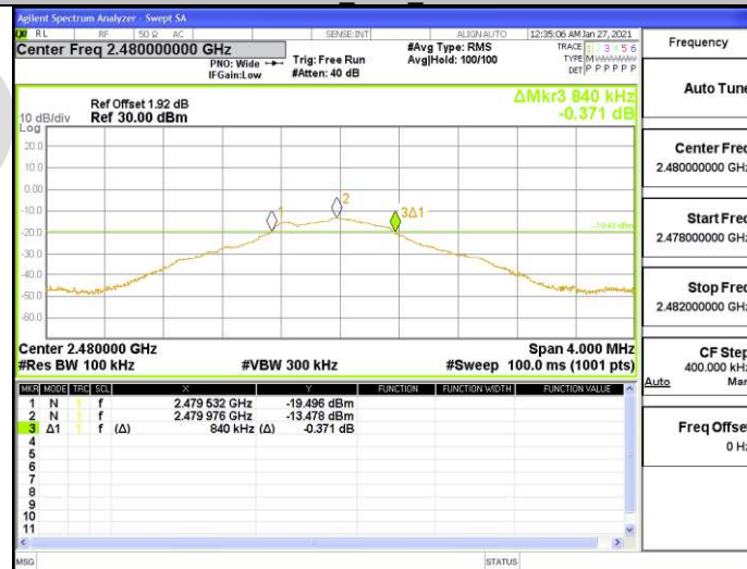
BLE Ant1 2480
