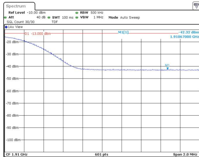
Band2-20MHz-16QAM-19100-1RB#99
