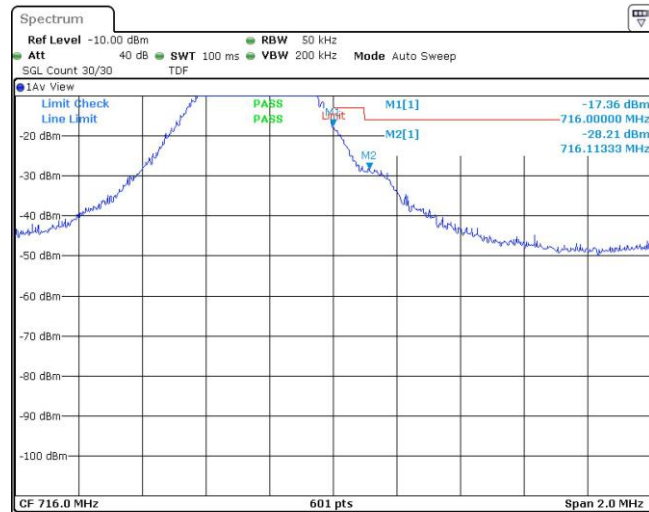
Band12-3MHz-QPSK-23165-15RB#0
