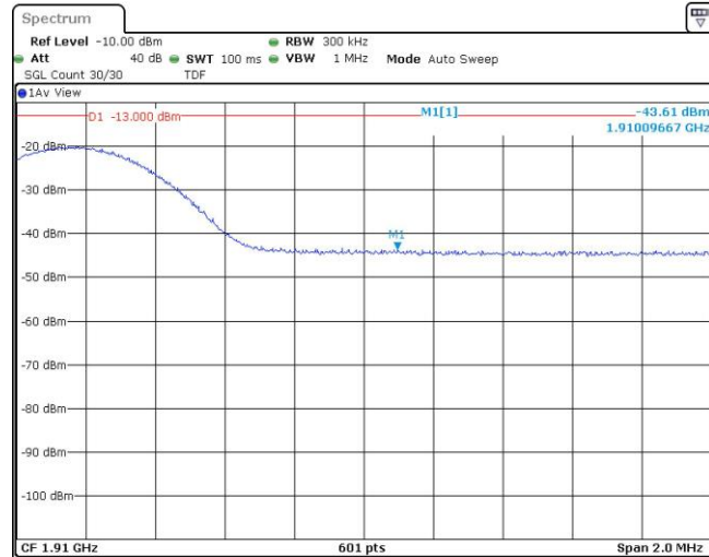
Band2-15MHz-16QAM-19125-1RB#74
