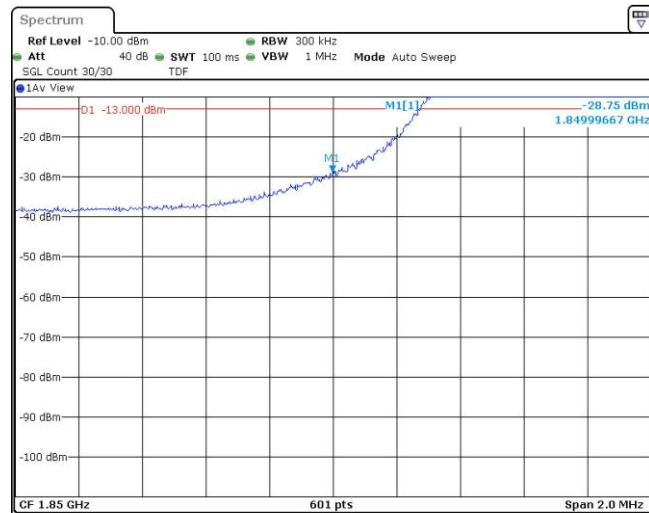
Band2-15MHz-16QAM-18675-1RB#74
