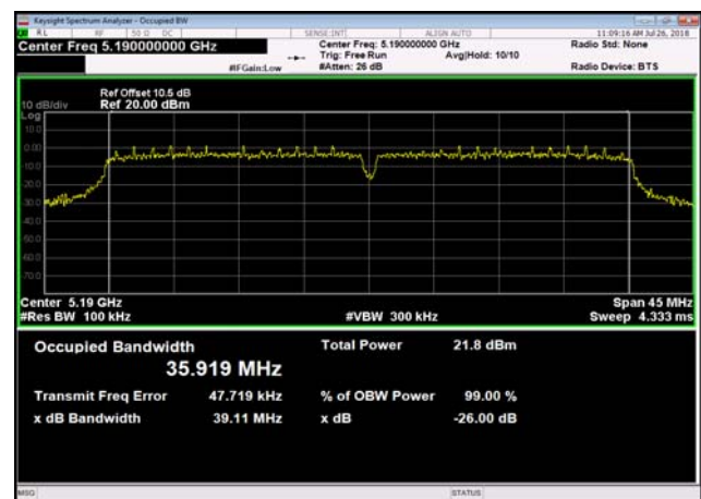
U-NII-1 26 dB Bandwidth-802.11ac(40MHz) ,5190MHz
