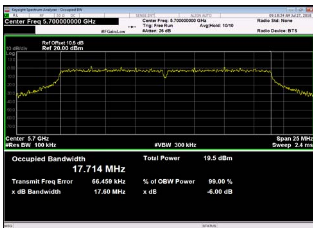
U-NII-2c 6dB Bandwidth-802.11n(20MHz) ,5700MHz
