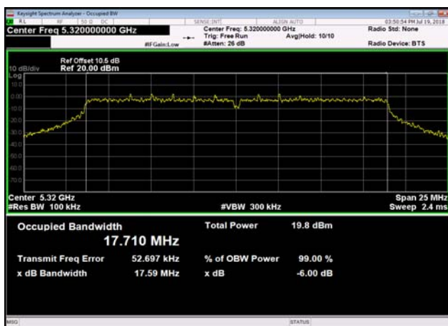
U-NII-2a 6dB Bandwidth-802.11ac(20MHz) ,5320MHz
