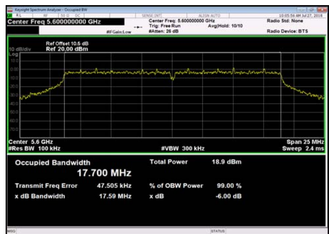
U-NII-2c 6dB Bandwidth-802.11ac(20MHz) ,5600MHz
