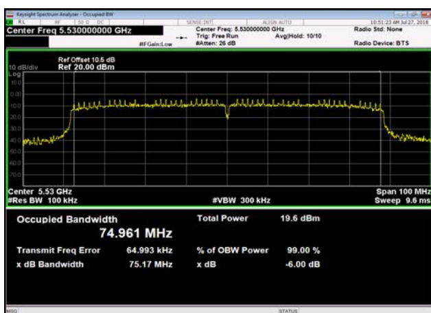
U-NII-2c 6dB Bandwidth-802.11ac(80MHz ) ,5530MHz
