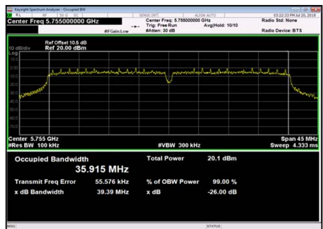
U-NII-3 26 dB Bandwidth-802.11ac(40MHz) ,5755MHz
