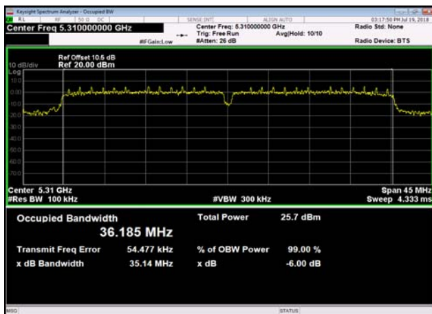
U-NII-2a 6dB Bandwidth-802.11ac(40MHz) ,5310MHz
