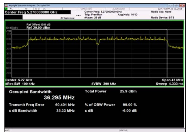
U-NII-2a 6dB Bandwidth-802.11ac(40MHz) ,5270MHz
