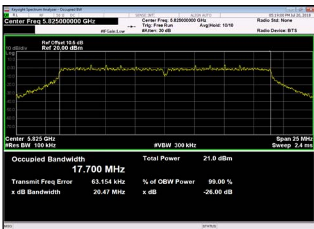
U-NII-3 26 dB Bandwidth-802.11ac(20MHz) ,5825MHz
