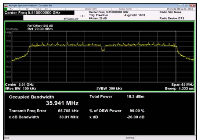
U-NII-2c 26 dB Bandwidth-802.11n(40MHz) ) ,5510MHz
