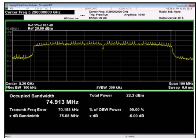
U-NII-2a 6dB Bandwidth-802.11ac(80MHz) ,5290MHz
