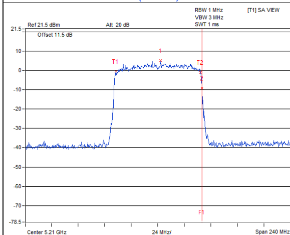
802.11ax (HE80+80) / Chain 0 : CH 42
