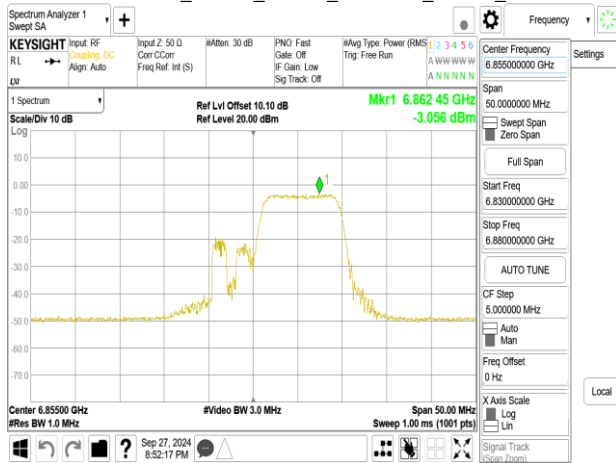
802.11be_20MHz_Chain1_6855MHz_RU26_8
