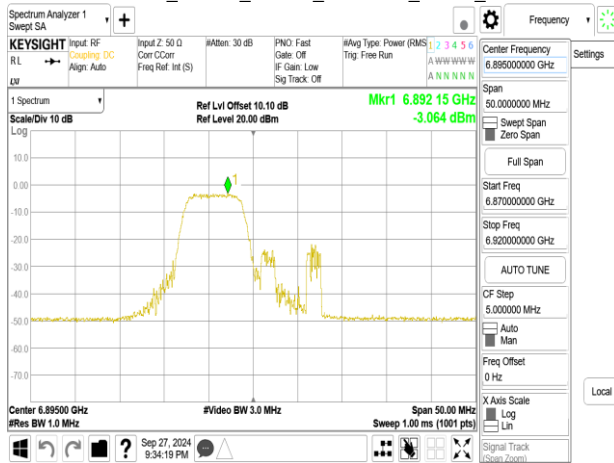
802.11be_20MHz_Chain1_6895MHz_RU106_53
