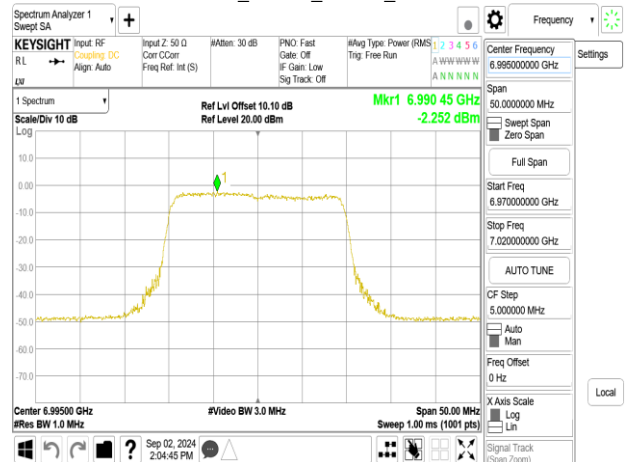
802.11be_20MHz_Chain1_6995MHz
