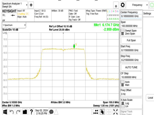
802.11be_40MHz_Chain1_6165MHz
