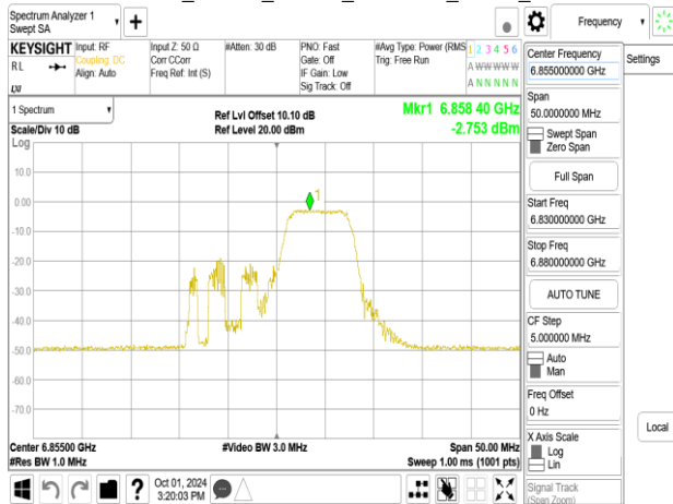
802.11be_20MHz_Chain1_6855MHz_RU106_54
