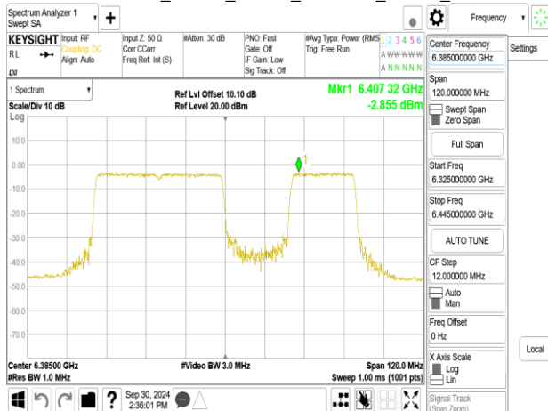
802.11be_80MHz_Chain0_6385MHz_RU484_66
