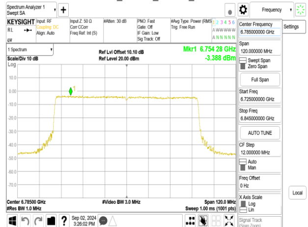
802.11be_80MHz_Chain0_6785MHz
