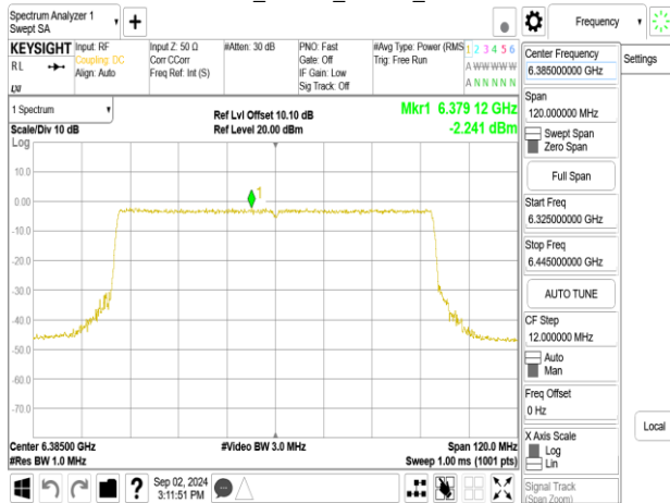
802.11be_80MHz_Chain0_6385MHz_484+242_MRU1
