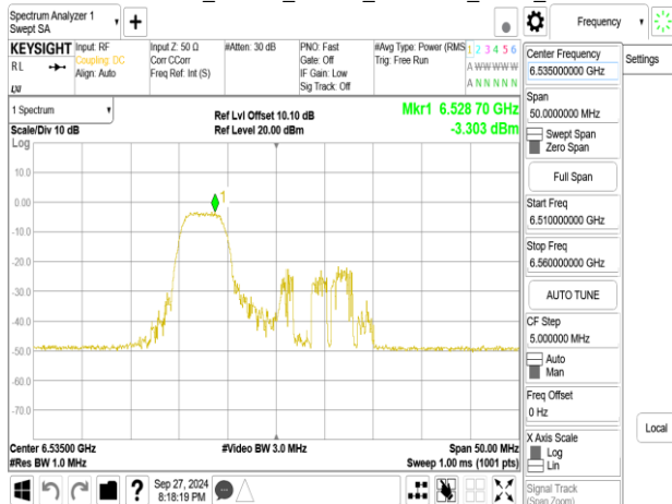
802.11be_20MHz_Chain1_6535MHz_RU52_37
