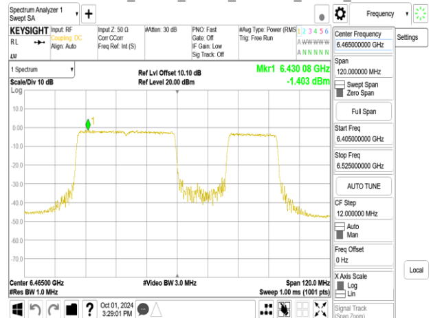
802.11be_80MHz_Chain0_6465MHz_RU484_65
