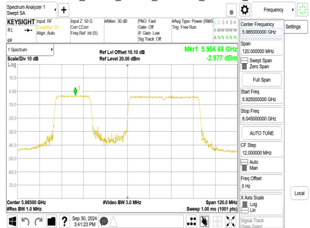
802.11be_80MHz_Chain0_5985MHz_RU484_65
