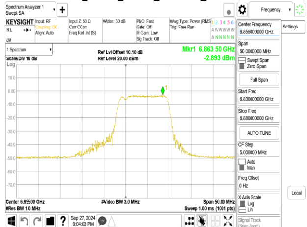
802.11be_20MHz_Chain1_6855MHz_106+26 MRU2
