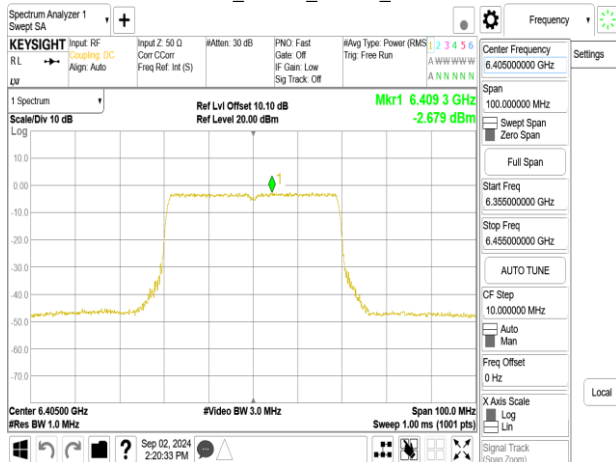
802.11be_40MHz_Chain0_6405MHz
