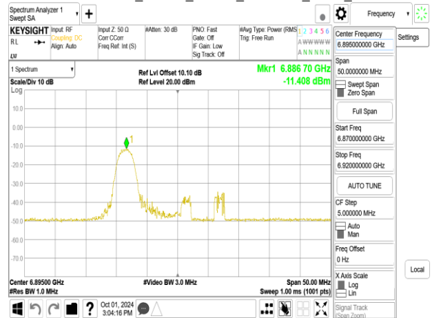
802.11be_20MHz_Chain1_6895MHz_RU52_37
