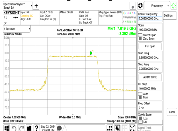
802.11be_40MHz_Chain0_7005MHz
