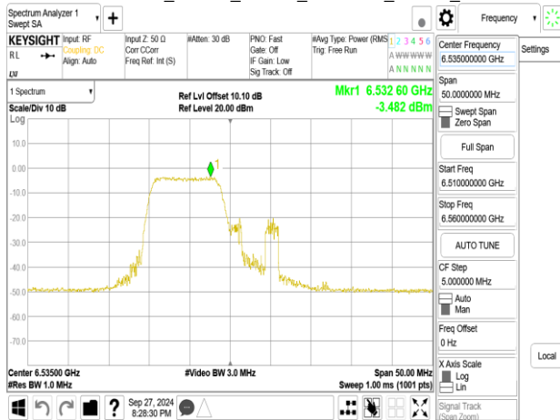
802.11be_20MHz_Chain1_6535MHz_RU26_0
