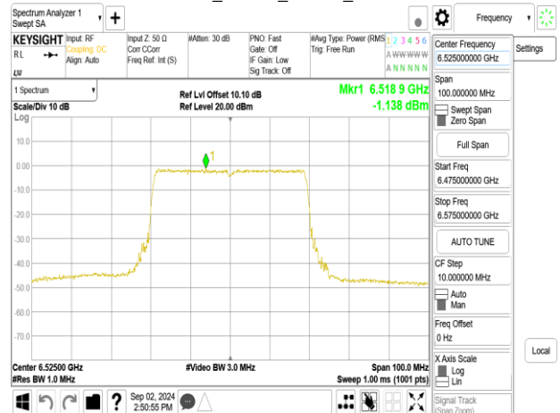
802.11be_40MHz_Chain0_6525MHz
