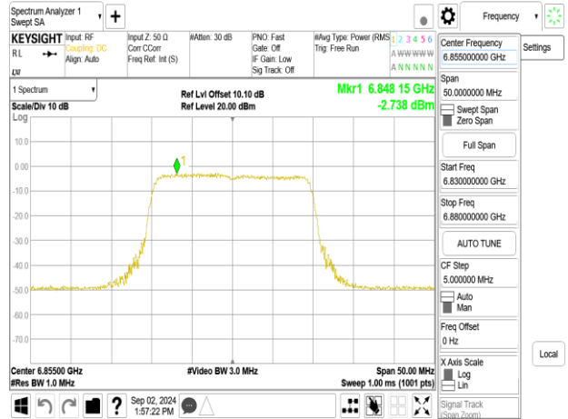
802.11be_20MHz_Chain1_6855MHz_106+26 MRU2
