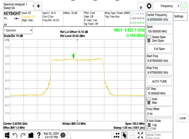
802.11be_40MHz_Chain1_6925MHz
