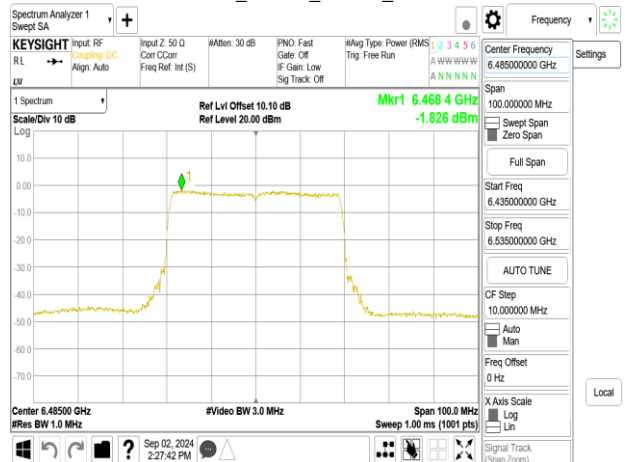
802.11be_40MHz_Chain1_6485MHz
