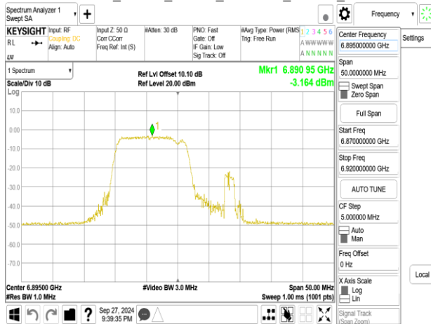
802.11be_20MHz_Chain1_6895MHz_52+26_MRU1
