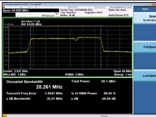
FDD7_MidRange_20+10_QPSK
