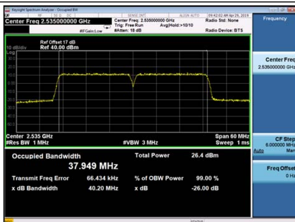
FDD7_MidRange_20+20_QPSK
