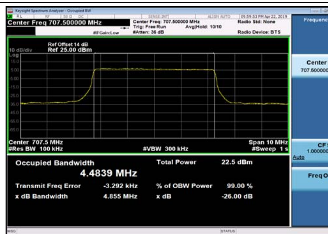
FDD12_MidRange_10MHz_707.5MHz_QPSK
