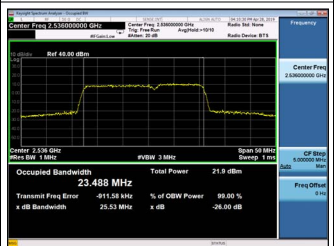
FDD7_MidRange_15+10_Q16
