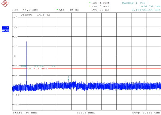
5MHz_Middle_QPSK_25@0 -24.76 dBm
