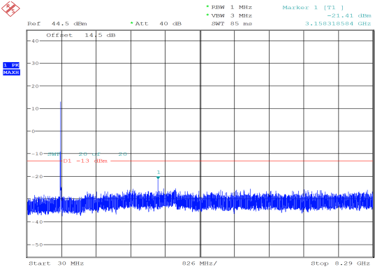
10MHz_Low_QPSK_50@0 -21.41 dBm
