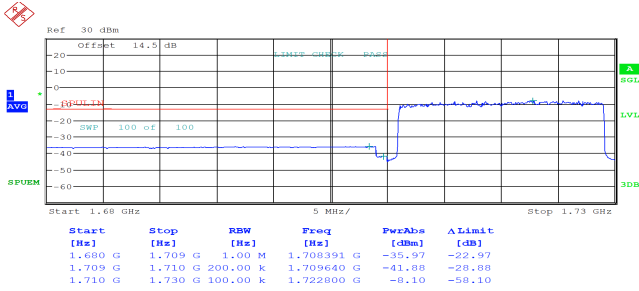
20MHz_Low_QPSK_100@0
