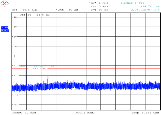
10MHz_Middle_QPSK_50@0 -24.74 dBm
