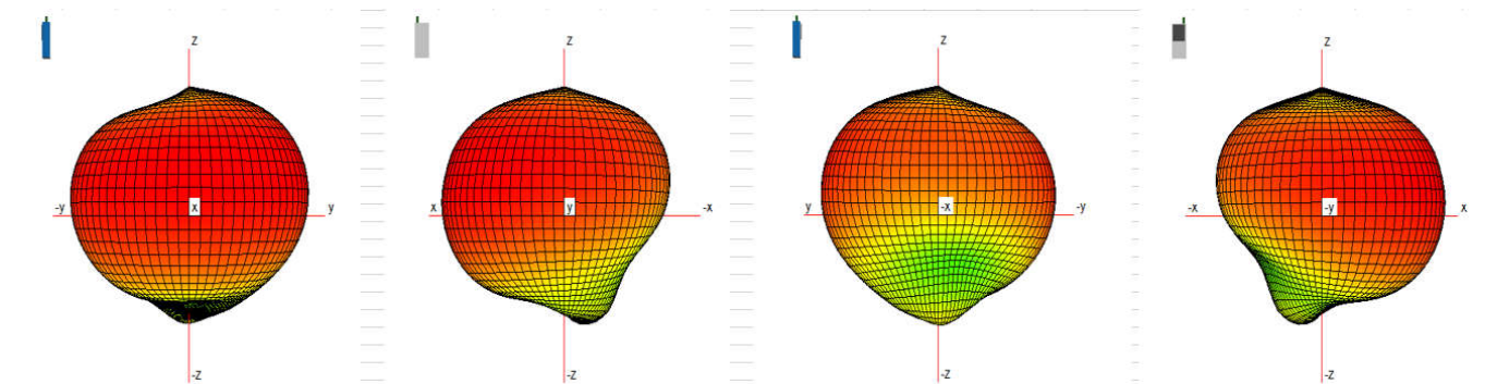
LTE B12
