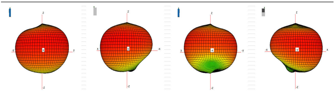
LTE B7
