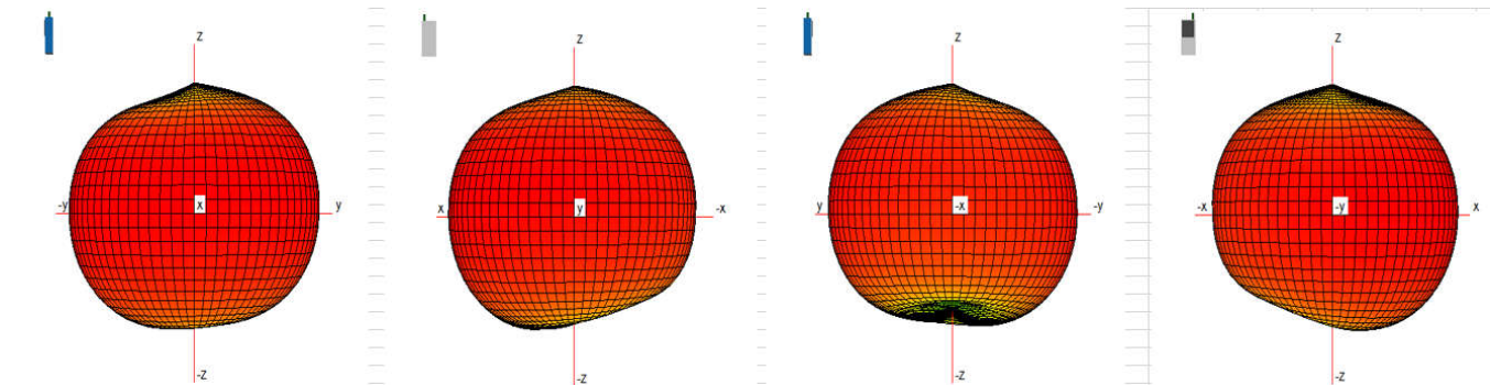
LTE B13
