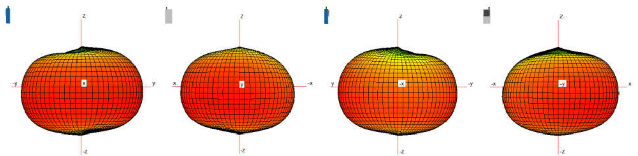
LTE B12
