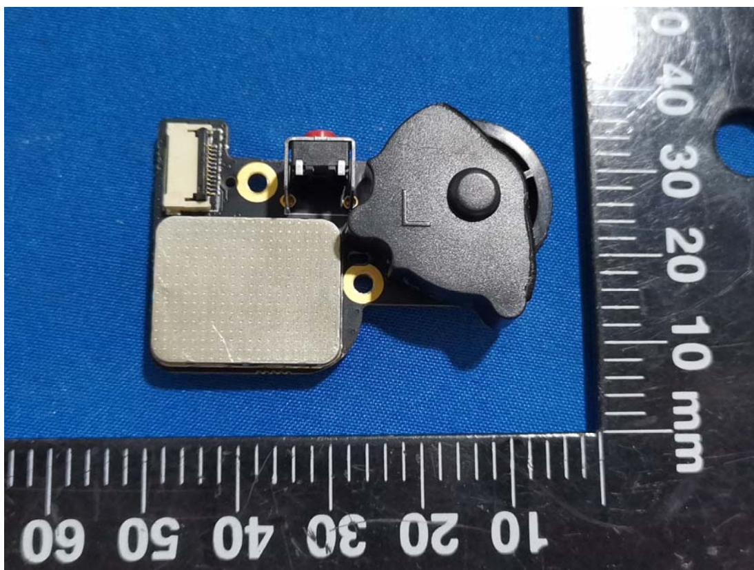
GPS Module
