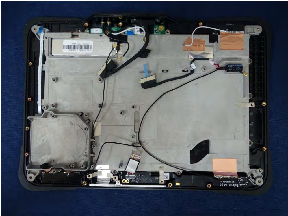
(95) EUT Photo
