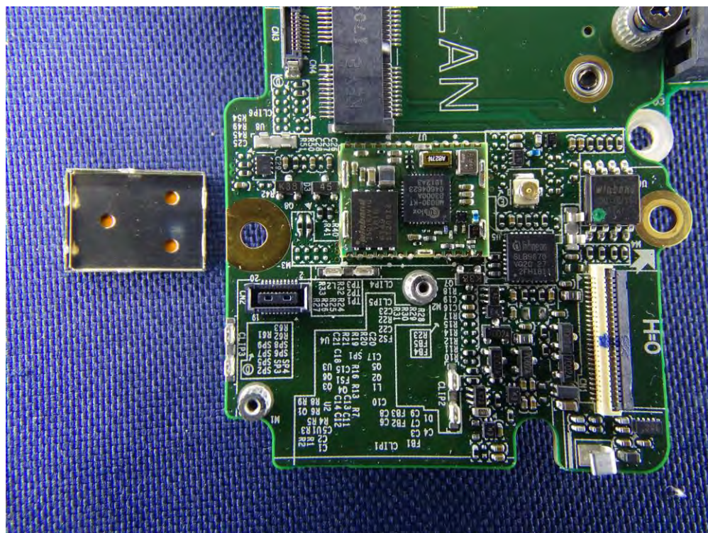
(72) EUT Photo
