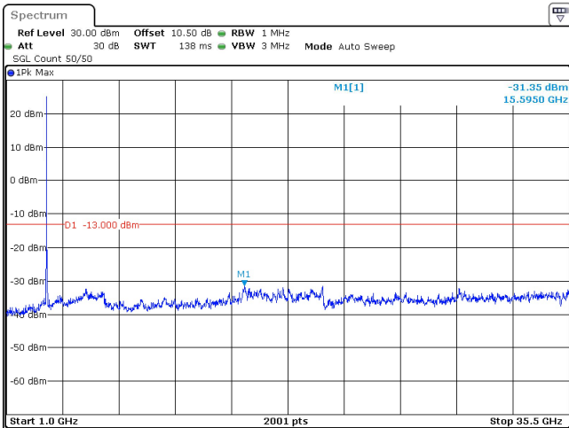
40MHz_30kHz_3470MHz_DFT-s-OFDM QPSK_RB1@0 -31.35 dBm
