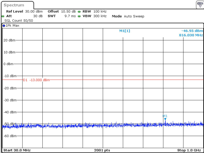
30MHz_30kHz_3535MHz_DFT-s-OFDM QPSK_RB1@77 -46.95 dBm
