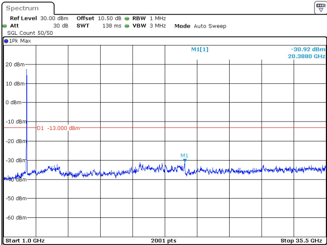
40MHz_30kHz_3470MHz_DFT-s-OFDM QPSK_RB100@0 -30.92 dBm
