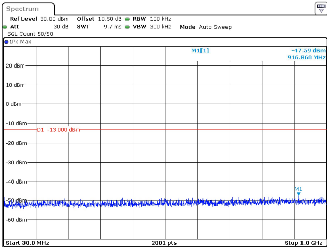
40MHz_30kHz_3530MHz_DFT-s-OFDM QPSK_RB1@0 -47.59 dBm
