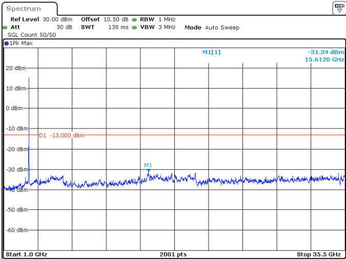
30MHz_30kHz_3535MHz_DFT-s-OFDM QPSK_RB75@0 -31.34 dBm
