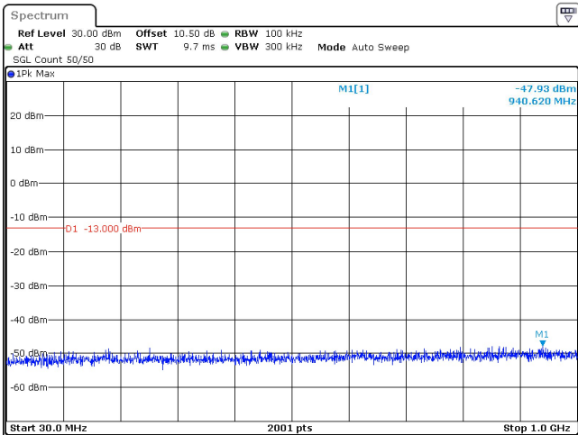
40MHz_30kHz_3470MHz_DFT-s-OFDM QPSK_RB1@0 -47.93 dBm
