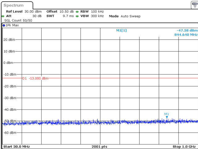
40MHz_30kHz_3500MHz_DFT-s-OFDM QPSK_RB1@0 -47.58 dBm
