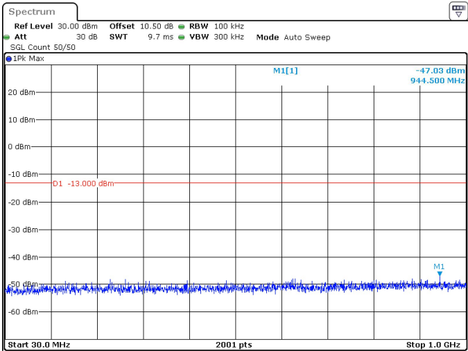
40MHz_30kHz_3470MHz_DFT-s-OFDM QPSK_RB100@0 -47.03 dBm
