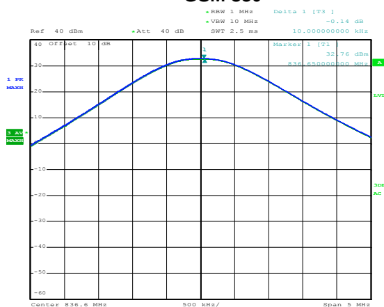
GSM 850
