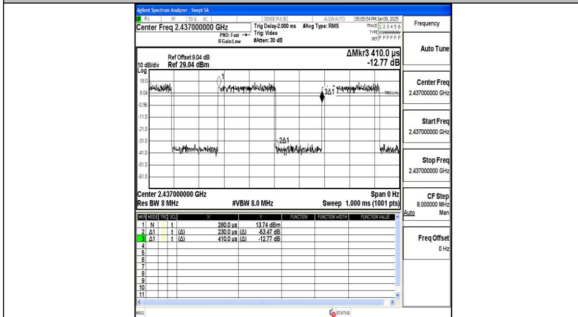
NTNV-11N20MIMO-Ant2-2437
