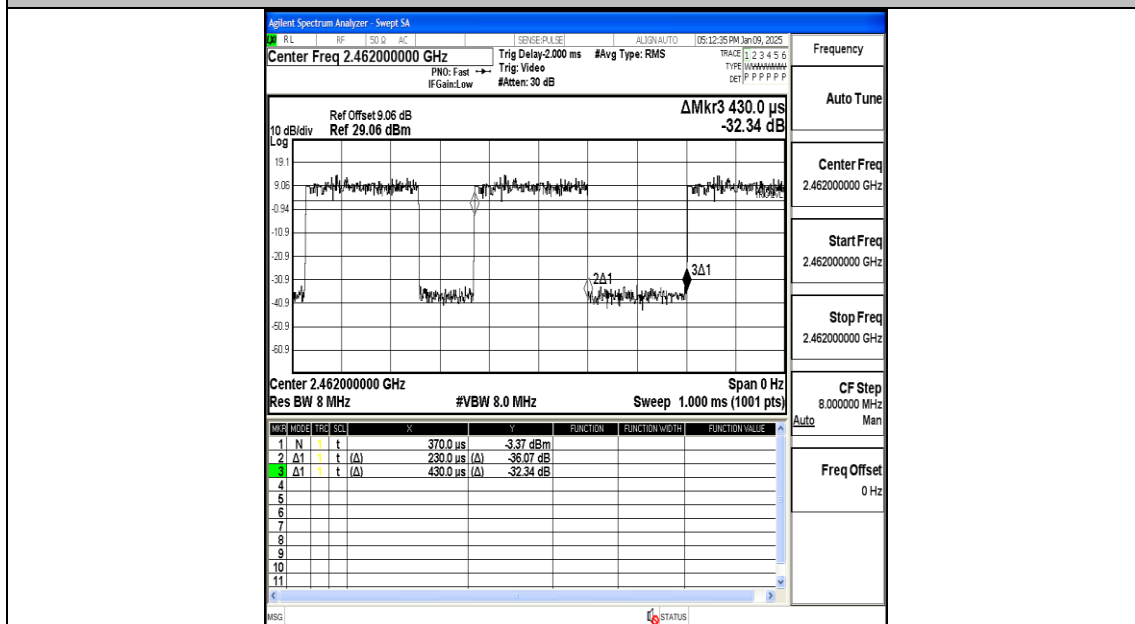
NTNV-11N20MIMO-Ant1-2462
