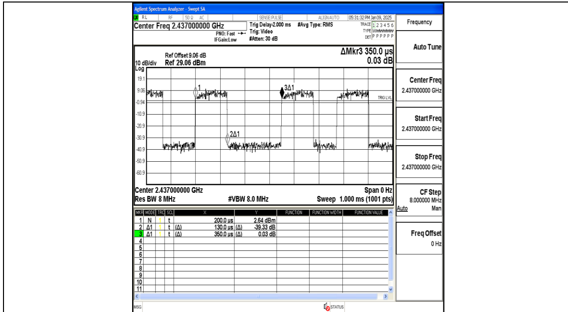
NTNV-11N40MIMO-Ant1-2437
