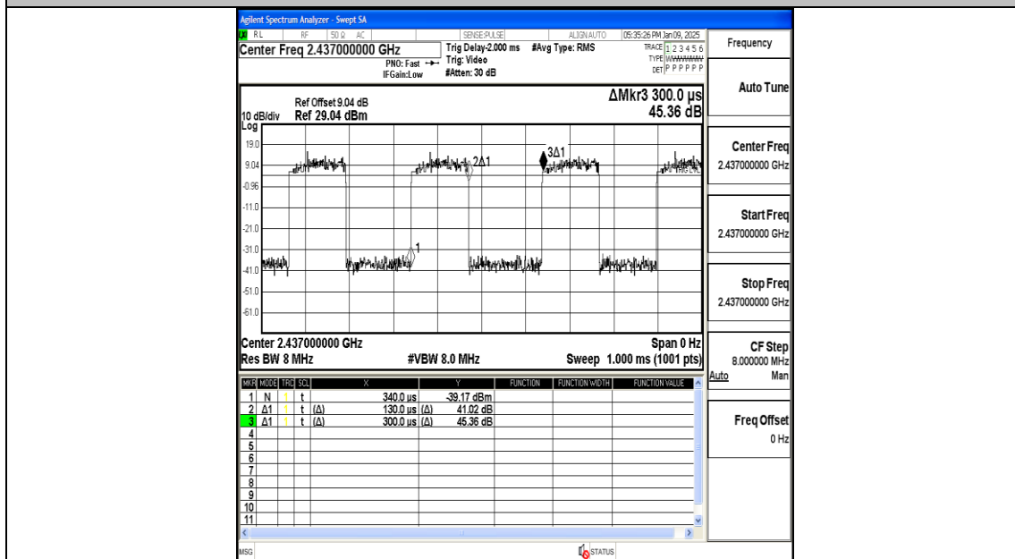
NTNV-11N40MIMO-Ant2-2437
