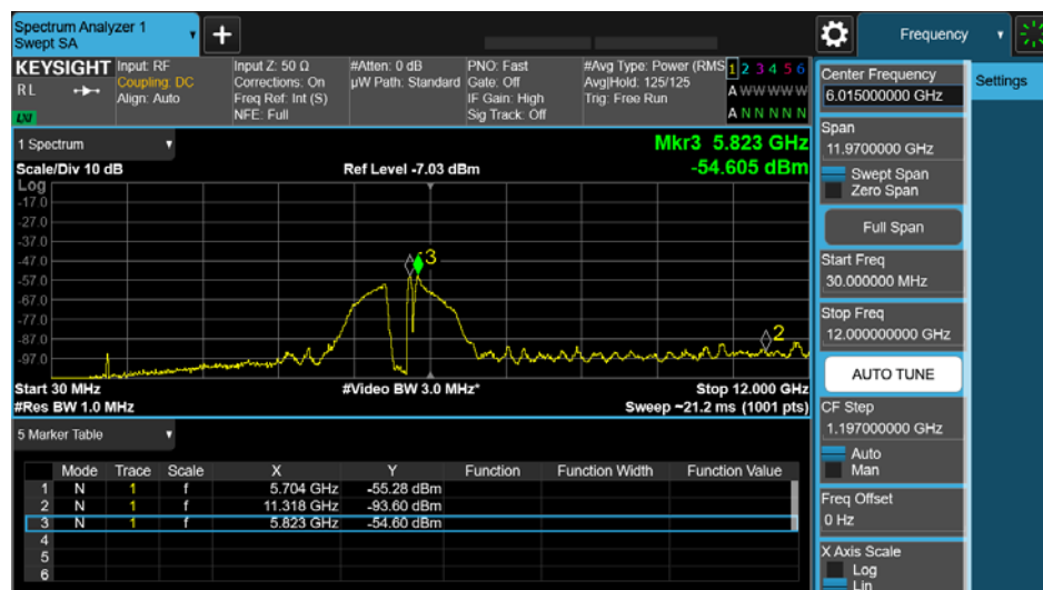
Antenna A
