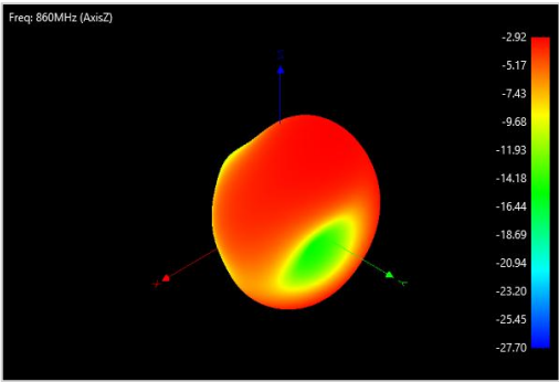
860.000Mhz
