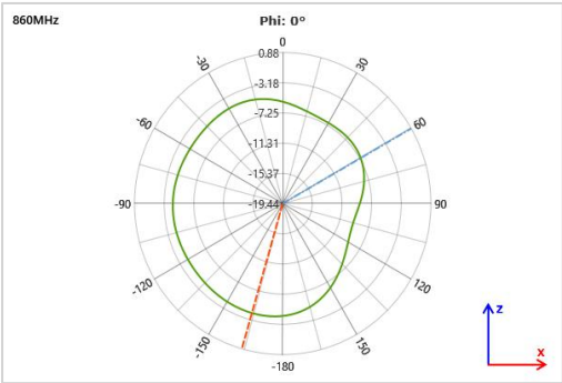
860.000Mhz E1
