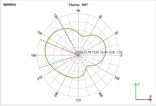
860.000Mhz E2
