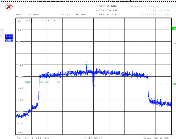
802.11ax(HT40)
