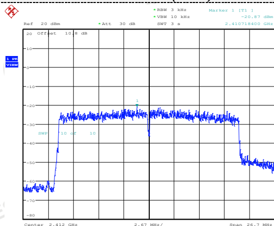
802.11ax(HT20)
