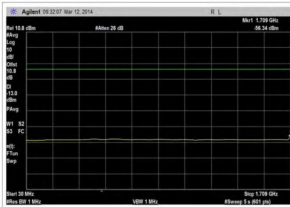
UL_1710-1755MHz_30-1709MHz
