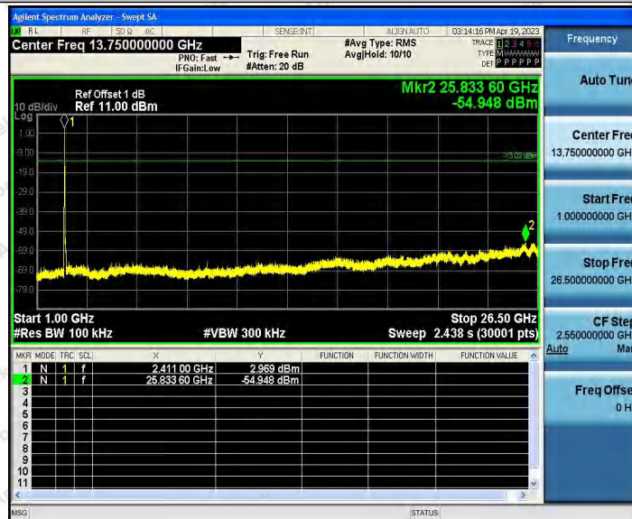
11N20_Ant2_2412_0~Reference
