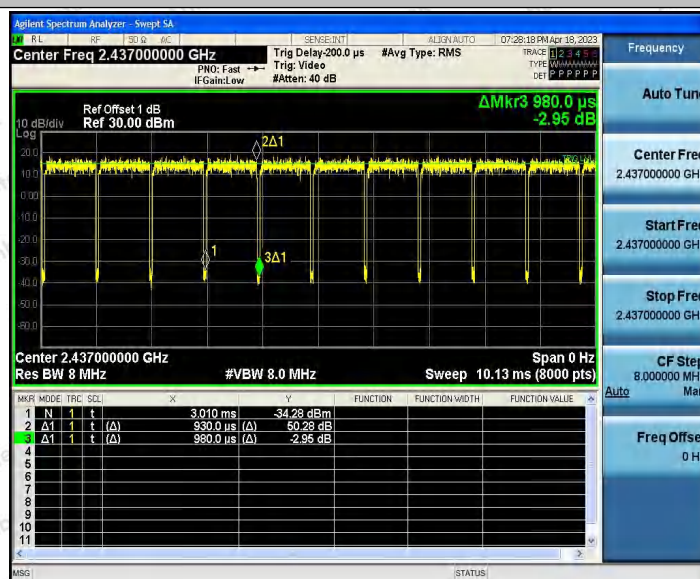
11N40_Ant2_2437
