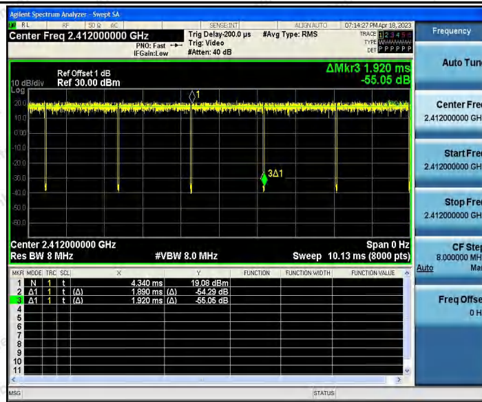
11N20_Ant2_2412
