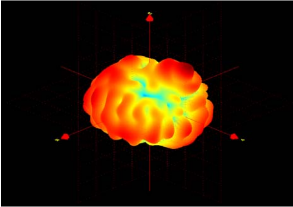
5180MHZ~5850MHZ(WIFI 5G)
