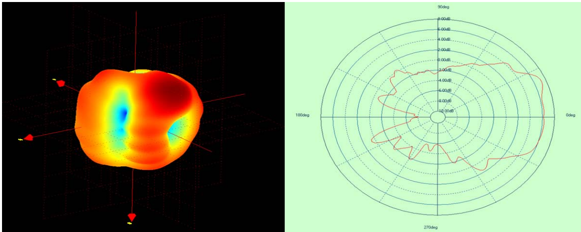
1550MHZ~1600MHZ(GPS)
