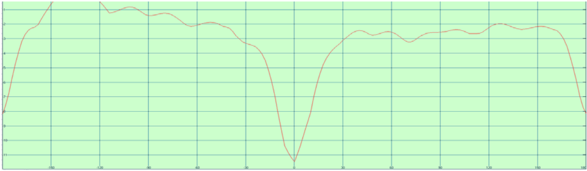
2400MHZ~2500MHZ(BT/WIFI 2.4G)
