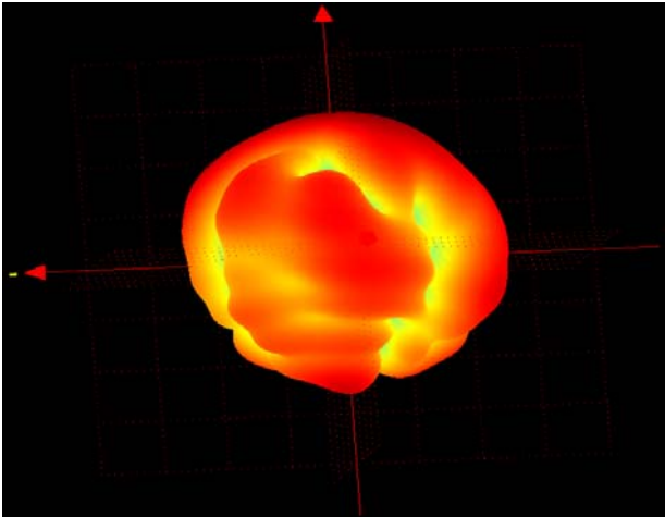
2400MHZ~2500MHZ(BT/WIFI 2.4G)
