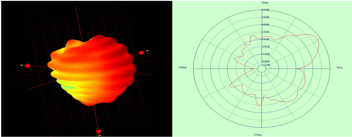
2500MHZ~2700MHZ
