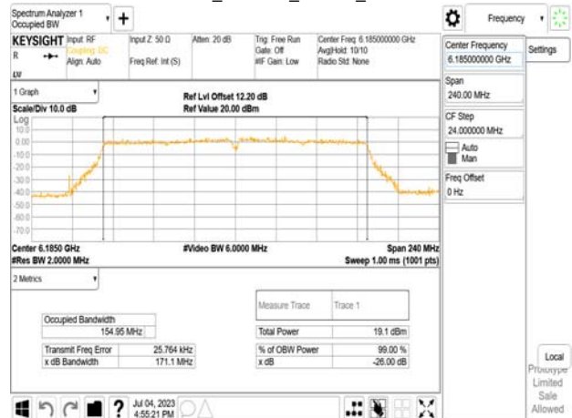
802.11ac_160MHz_Chain0_6185MHz
