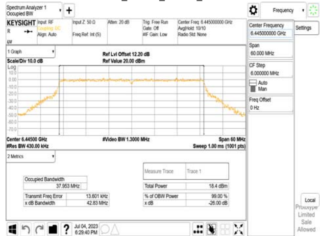
802.11be_40MHz_Chain0_6445MHz
