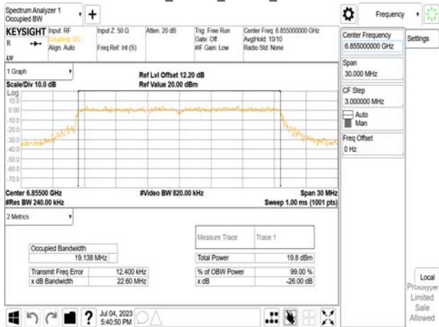
802.11be_20MHz_Chain0_6855MHz
