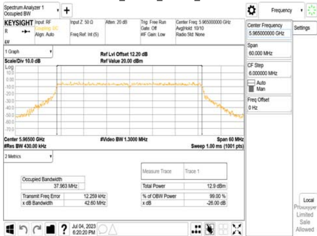
802.11be_40MHz_Chain0_5965MHz
