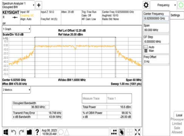
802.11n_40MHz_Chain0_6925MHz
