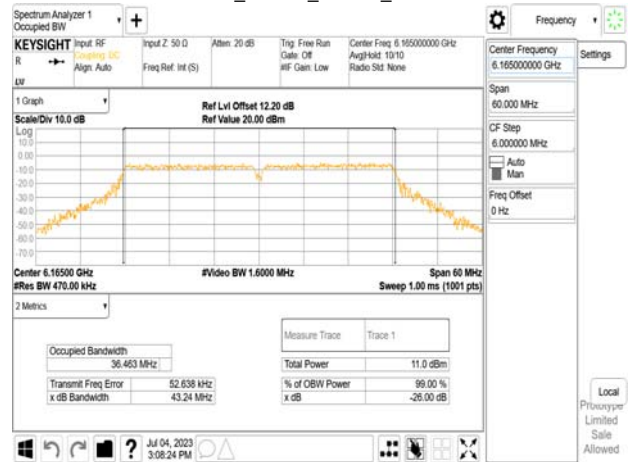
802.11n_40MHz_Chain0_6165MHz
