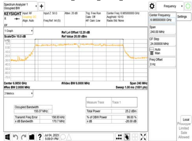
802.11ac_160MHz_Chain1_6985MHz
