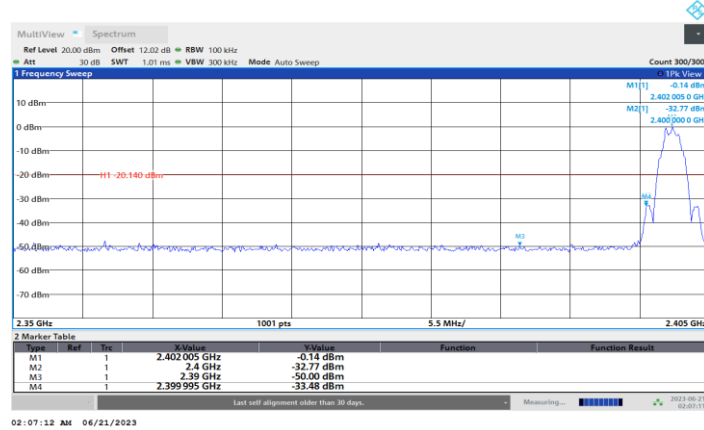
BLE_2M_Ant1_Low_2402
