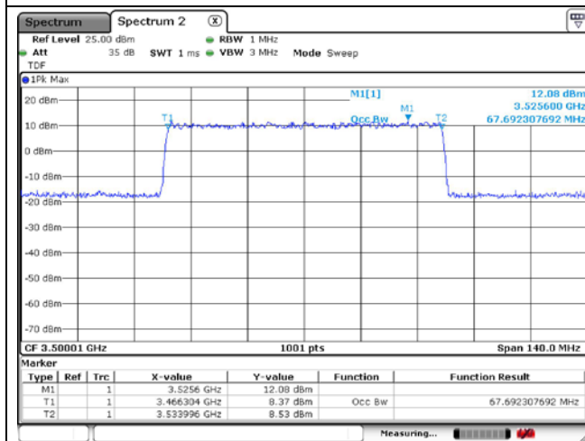
70 MHz CP-OFDM QPSK
