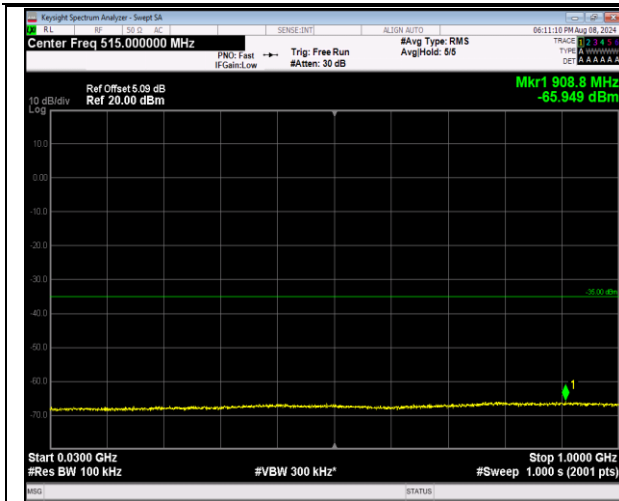
7-7-10MHz-20MHz-QPSK-QPSK-20805-20949-1RB#0-0 RB#0-30~1000MHz-PASS
