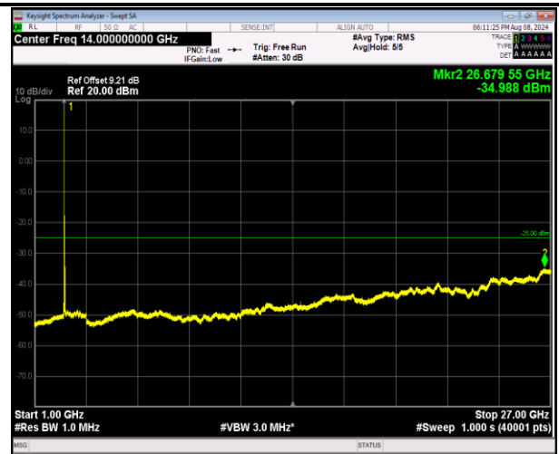
7-7-10MHz-20MHz-QPSK-QPSK-20805-20949-1RB#0-0 RB#0-1000~27000MHz-PASS
