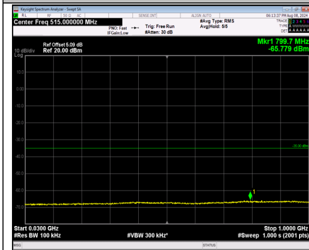
7-7-10MHz-20MHz-QPSK-QPSK-20805-20949-1RB#0-1 RB#99-30~1000MHz-PASS
