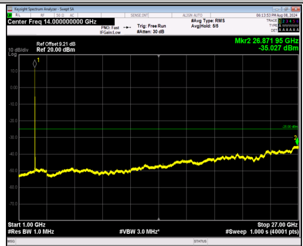
7-7-10MHz-20MHz-QPSK-QPSK-20805-20949-1RB#0-1 RB#99-1000~27000MHz-PASS
