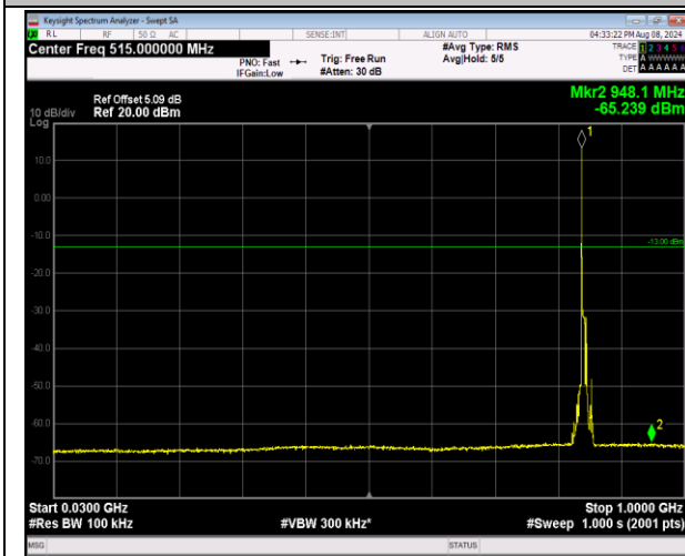
5-5-5MHz-3MHz-QPSK-QPSK-20595-20634-1RB#0-1R B#15-30~1000MHz-PASS
