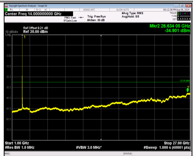
7-7-10MHz-20MHz-QPSK-QPSK-20805-20949-1RB#49-0 RB#0-1000~27000MHz-PASS
