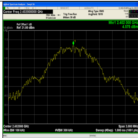
BLE 1M-Ant10-2402-0~Reference
