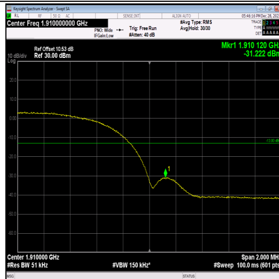
Band2-9538-3-PASS
