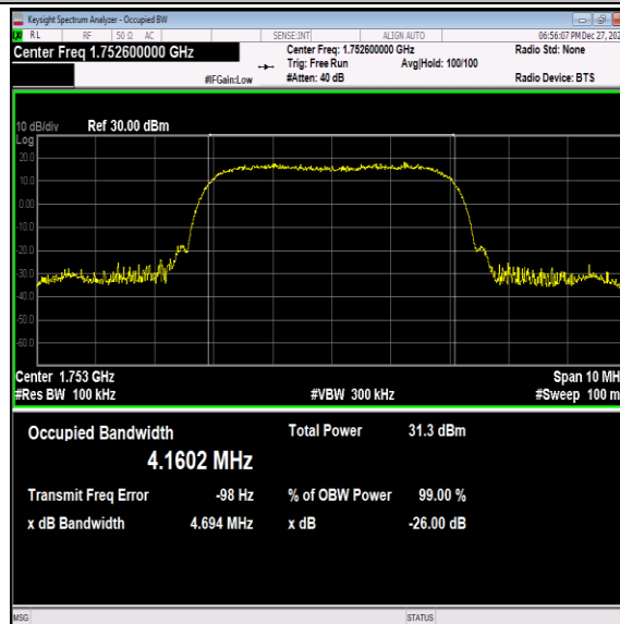
Band4-1513-5-PASS
