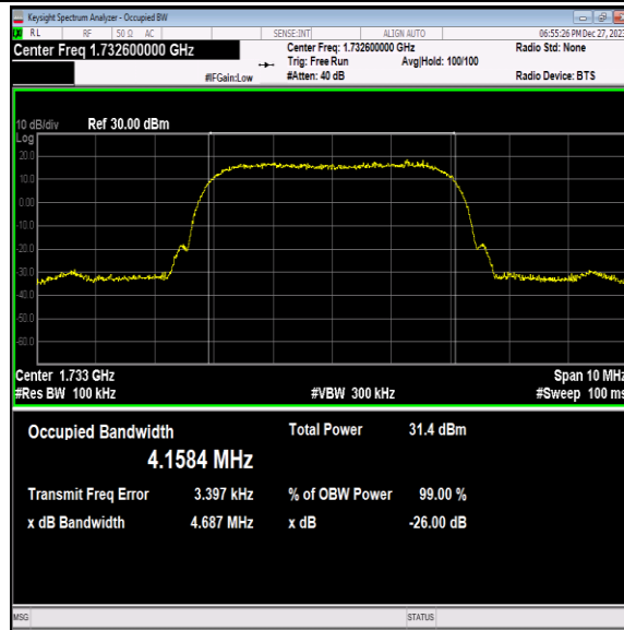
Band4-1413-5-PASS
