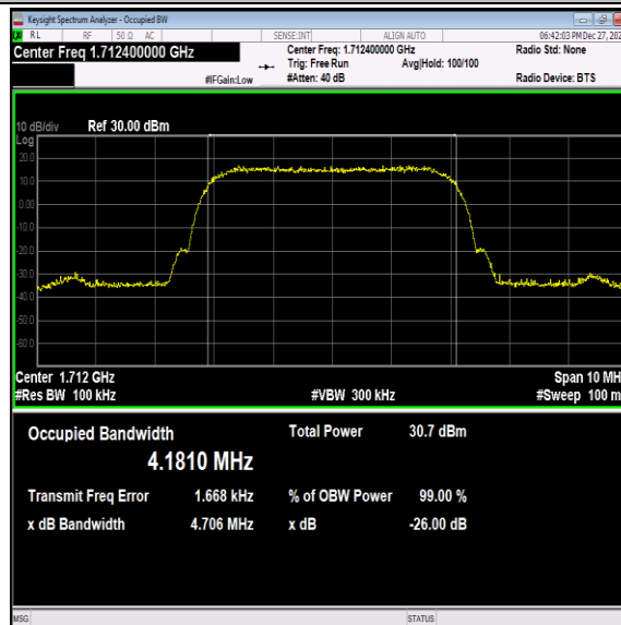
Band4-1312-1-PASS
