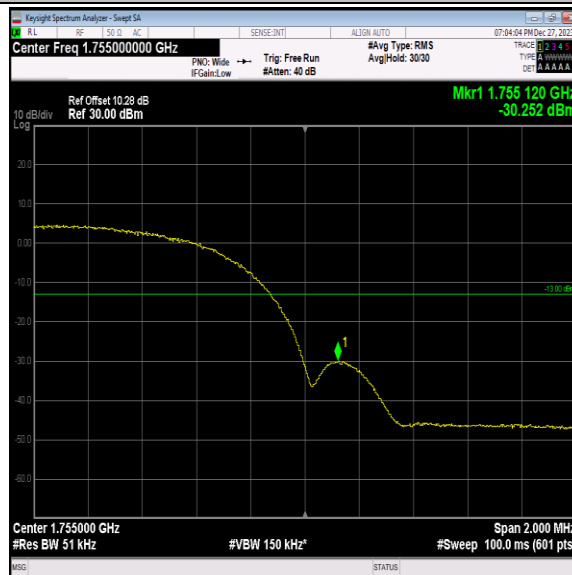
Band4-1513-5-PASS
