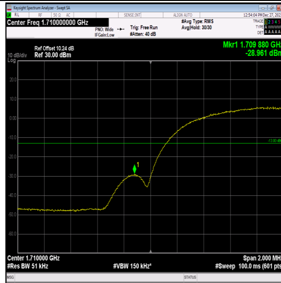
Band4-1312-1-PASS
