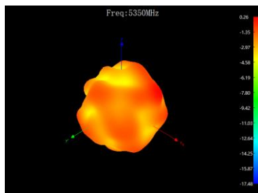
ZXY face @5350MHz
