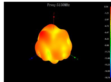
YZX face @5150MHz
