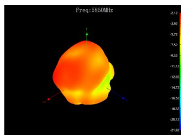
XYZ face @5850MHz
