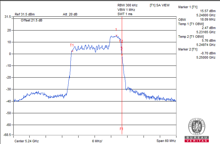
802.11ax (HE) 52-tone RU : CH 48
