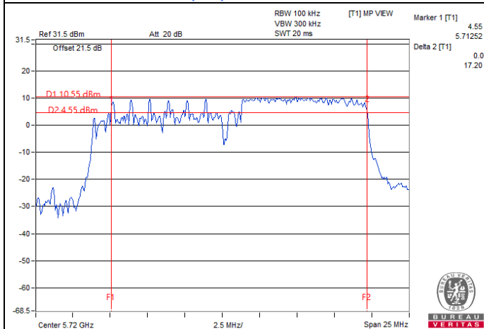
802.11ax (HE) 106-tone RU : CH 144 (U-NII-3)
