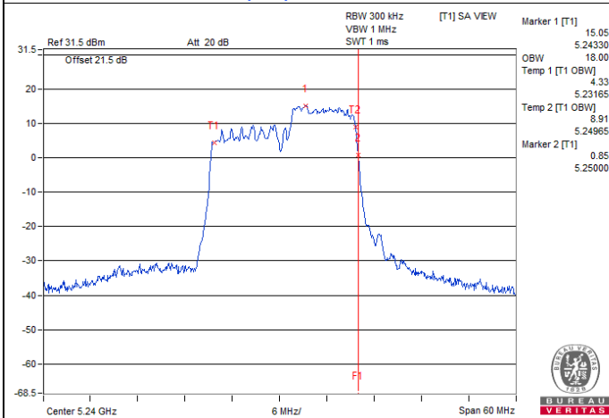
802.11ax (HE) 106-tone RU : CH 48
