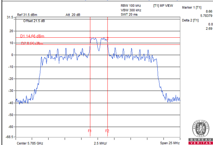
802.11ax (HE) 26-tone RU : CH 157
