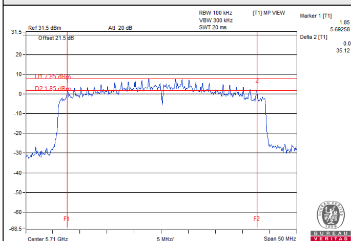
802.11ax (HE40) : CH 142 (U-NII-3)
