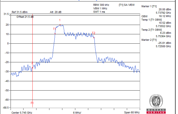
802.11ax (HE) 52-tone RU : CH 149
