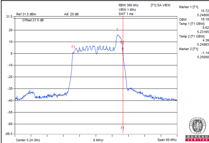
802.11ax (HE) 26-tone RU : CH 48
