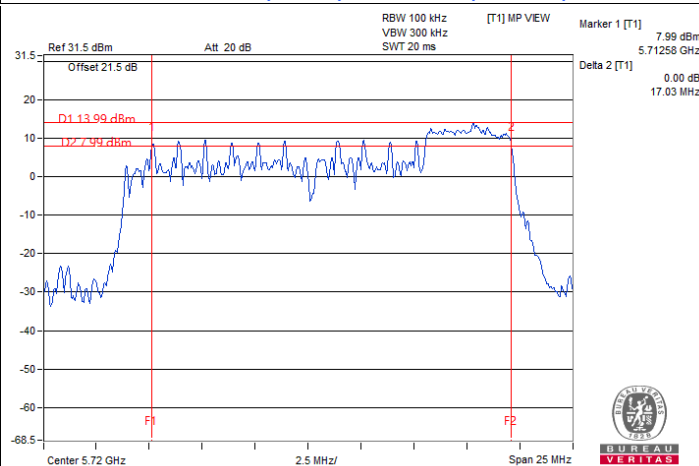
802.11ax (HE) 52-tone RU : CH 144 (U-NII-3)
