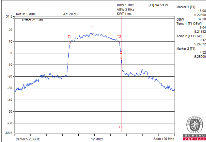
802.11ax (HE40) : CH 46
