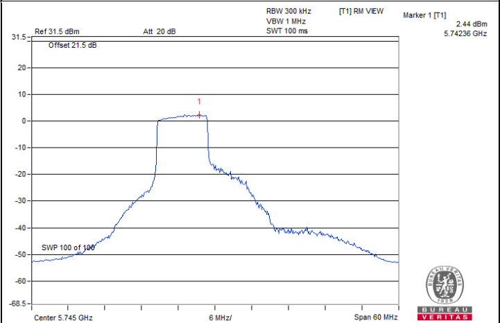
802.11ax (HE) 106-tone RU : CH 149
