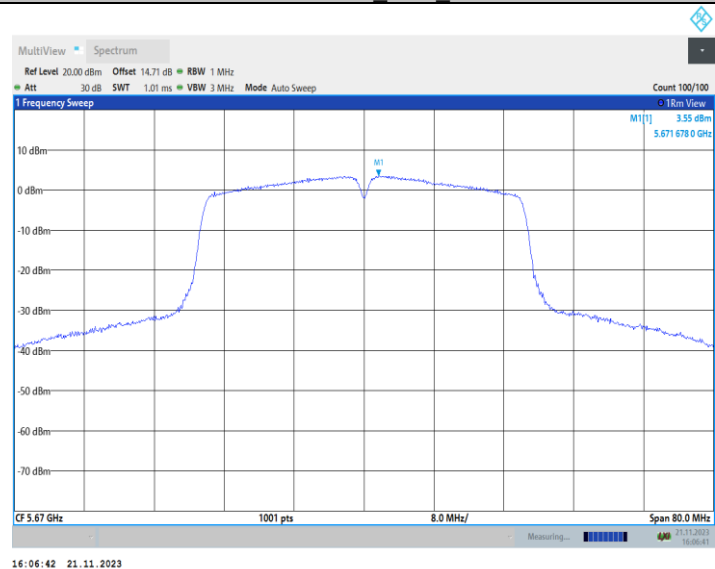
11AC40MIMO_Ant2_5670
