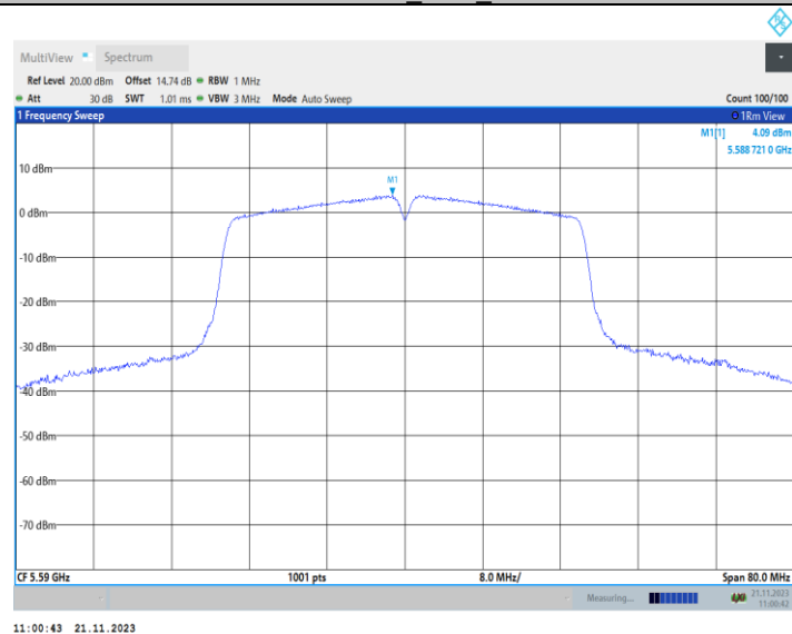
11N40MIMO_Ant2_5590
