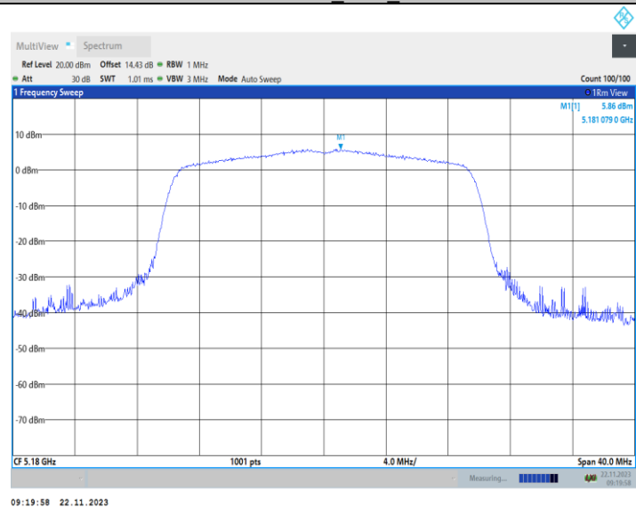
11AX20MIMO_Ant2_5180
