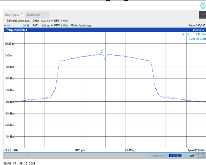
11N40MIMO_Ant2_5310
