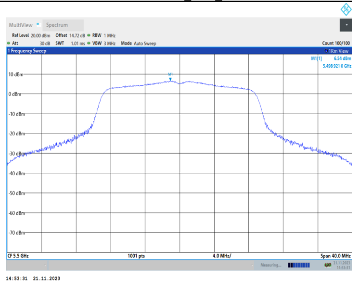
11AC20MIMO_Ant2_5500
