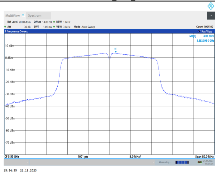
11AC40MIMO_Ant2_5590
