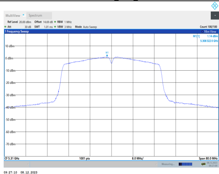
11AC40MIMO_Ant2_5310
