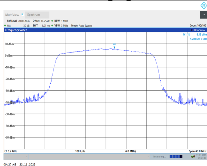
11AX20MIMO_Ant2_5200
