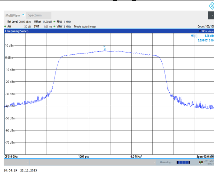
11AX20MIMO_Ant2_5600
