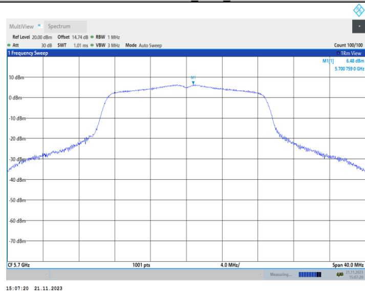
11AC20MIMO_Ant2_5700
