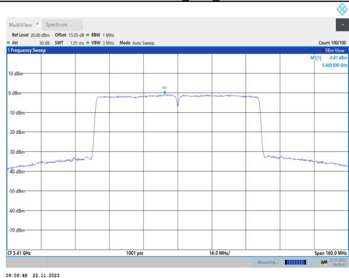
11AC80MIMO_Ant2_5610
