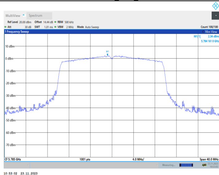
11AX20MIMO_Ant2_5785
