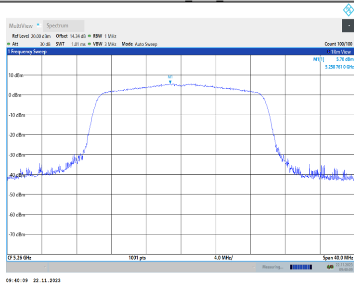
11AX20MIMO_Ant2_5260
