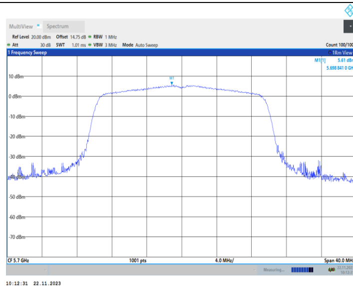
11AX20MIMO_Ant2_5700
