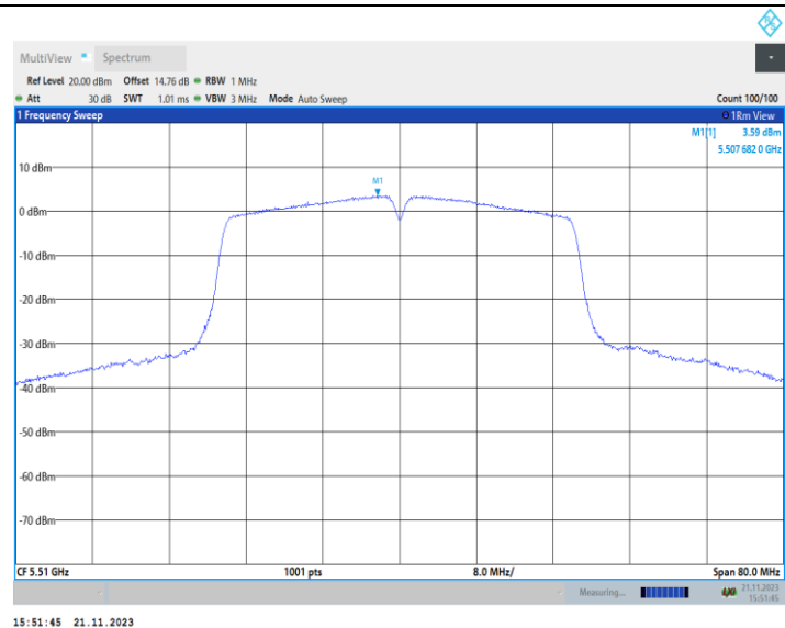
11AC40MIMO_Ant2_5510
