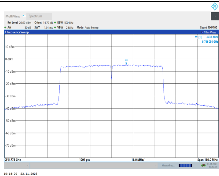
11AC80MIMO_Ant2_5775
