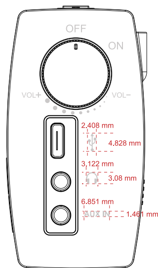
侧面丝印
