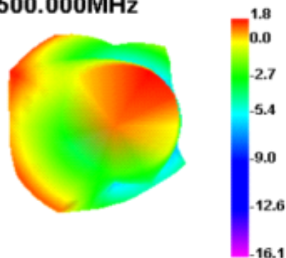
2500.000MHz E1
