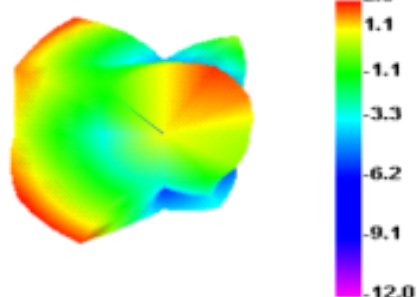
2450.000MHz E1
