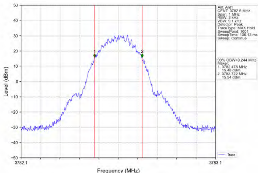
Bandn77a_3782.6MHz_GMSK_SISO_Ant1_NTNV_Output_AGC+3
