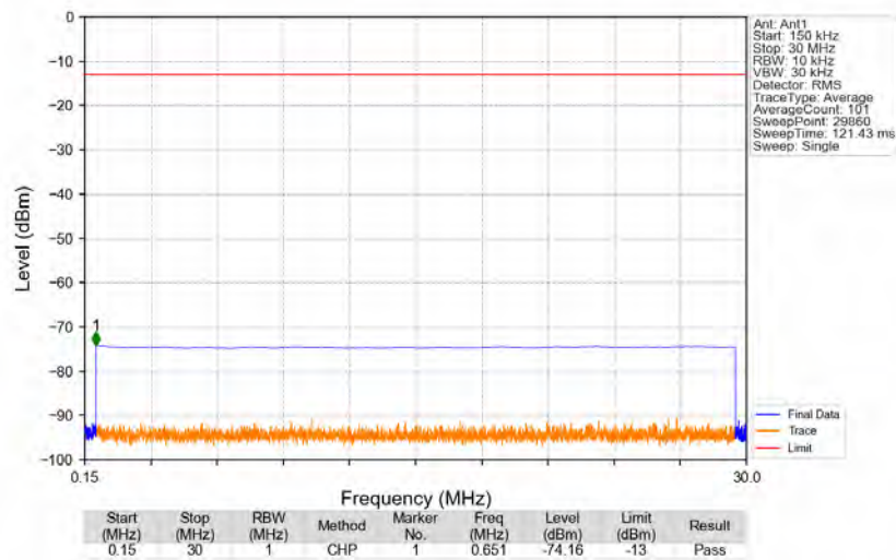
Bandn77a_3840MHz_GMSK_SISO_Ant1_NTNV
