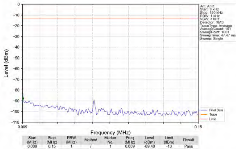
Bandn77a_3840MHz_GMSK_SISO_Ant1_NTNV
