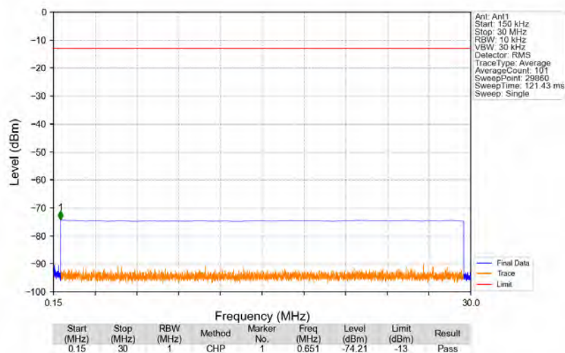
Bandn77a_3977.5MHz_AWGN_SISO_Ant1_NTNV
