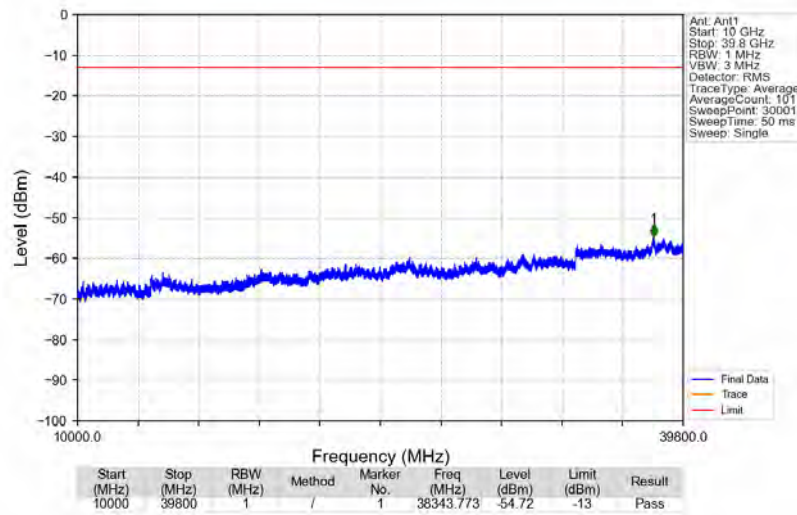
Bandn77a_3977.5MHz_AWGN_SISO_Ant1_NTNV
