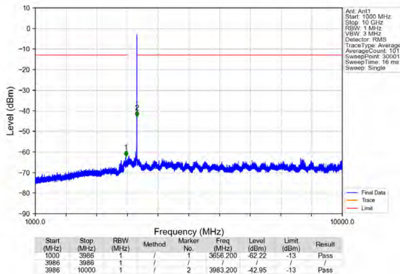
Bandn77a_3977.5MHz_AWGN_SISO_Ant1_NTNV
