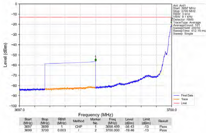
Bandn77a_3700.2MHz_GMSK_SISO_Ant1_NTNV_AGC+3
