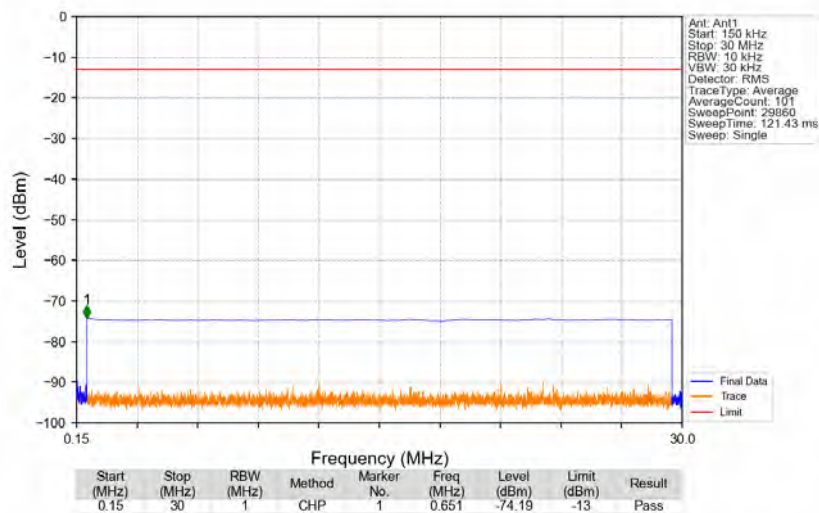
Bandn77a_3840MHz_AWGN_SISO_Ant1_NTNV
