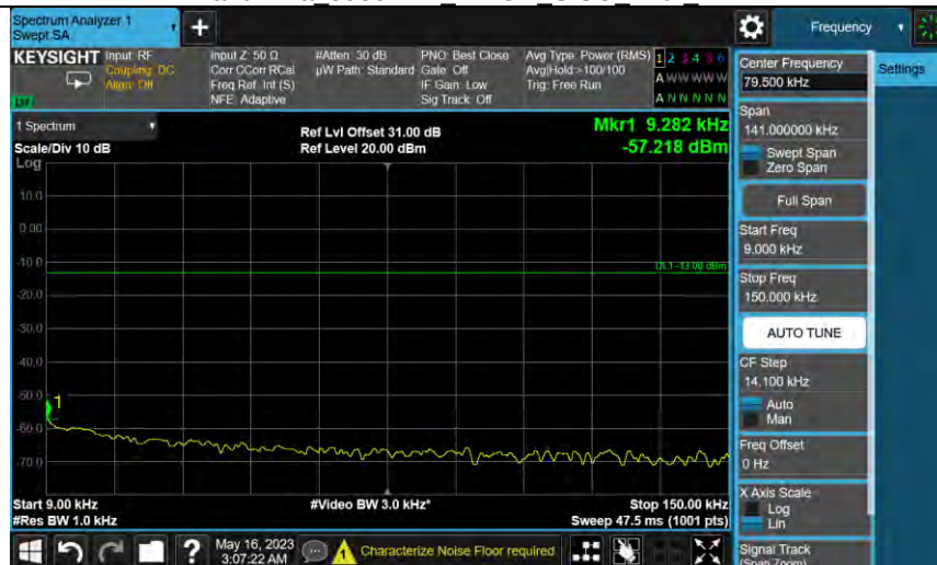
Bandn77a 3930MHz AWGN SISO Ant1 NTN
