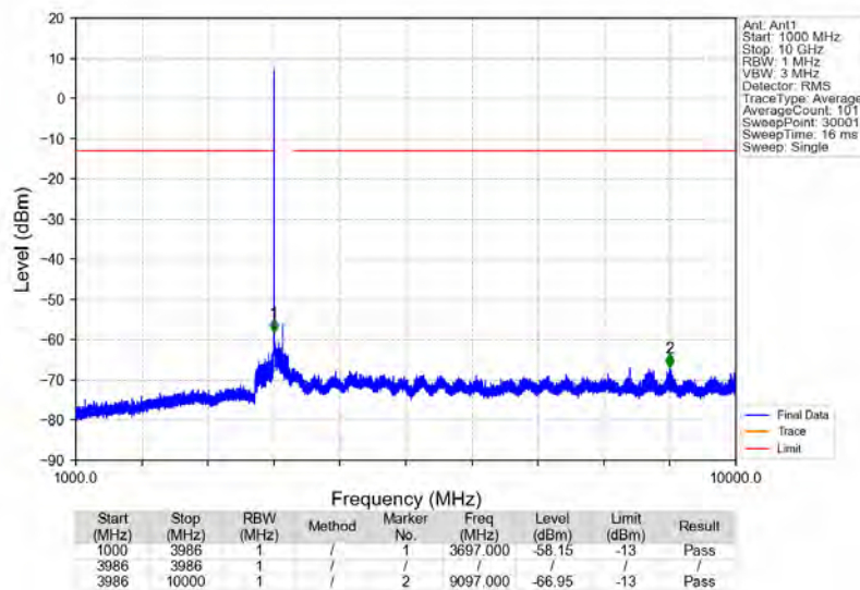
Bandn77a_3700.2MHz_GMSK_SISO_Ant1_NTNV
