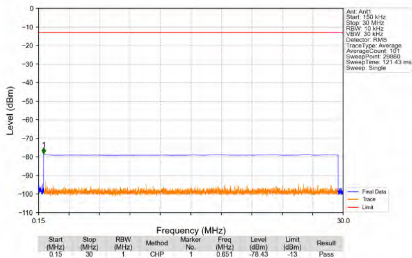
Bandn77a_3700.2MHz_GMSK_SISO_Ant1_NTNV
