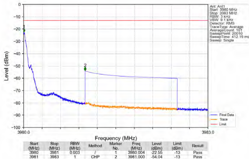
Bandn77a_3979.8MHz_GMSK_SISO_Ant1_NTNV_AGC
