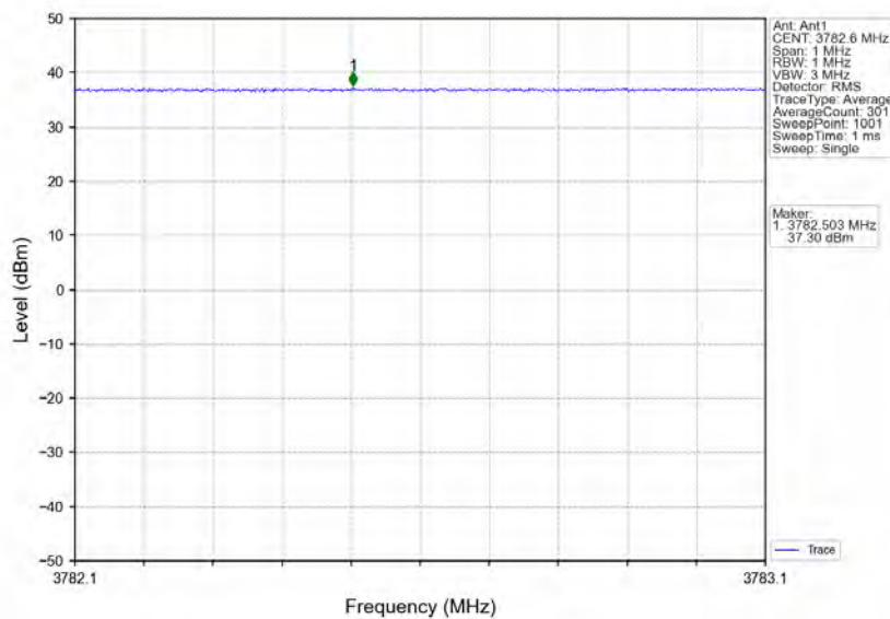
Bandn77a_3782.6MHz_GMSK_SISO_Ant1_NTNV_AGC+3
