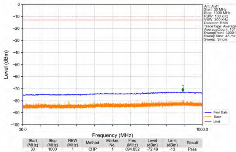
Bandn77a_3977.5MHz_AWGN_SISO_Ant1_NTNV
