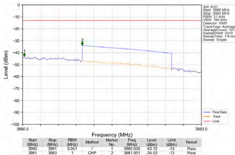
Bandn77a_3977.5MHz_AWGN_SISO_Ant1_NTNV_AGC
