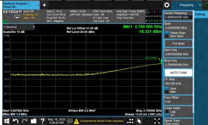
Bandn77a 3750MHz AWGN SISO Ant1 NTN AGC+3
