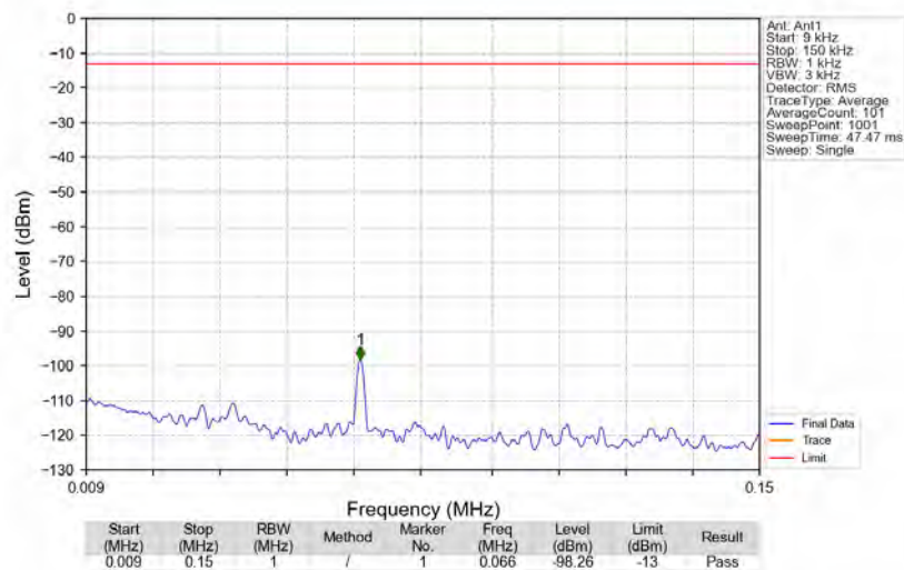
Bandn77a_3977.5MHz_AWGN_SISO_Ant1_NTNV
