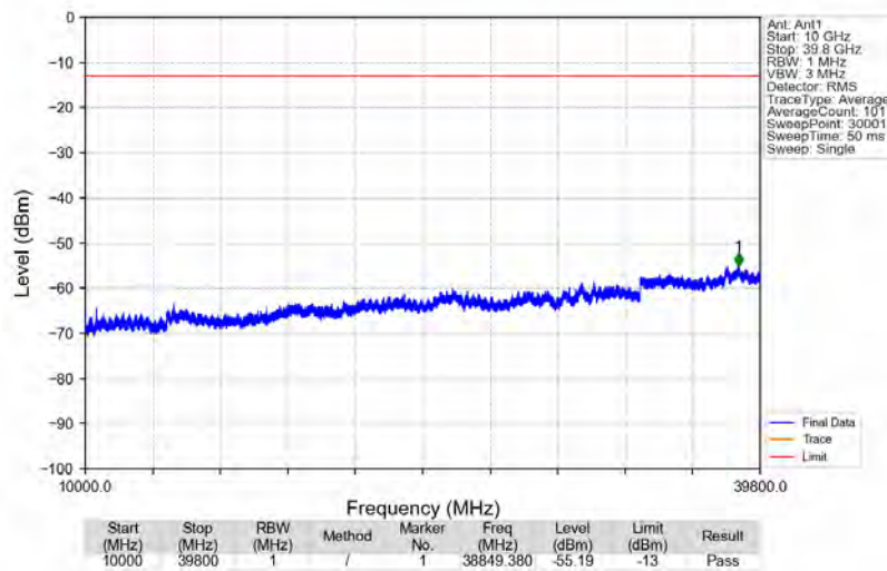
Bandn77a_3979.8MHz_GMSK_SISO_Ant1_NTNV
