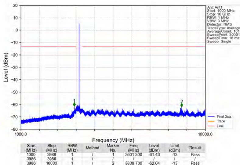
Bandn77a_3840MHz_GMSK_SISO_Ant1_NTNV
