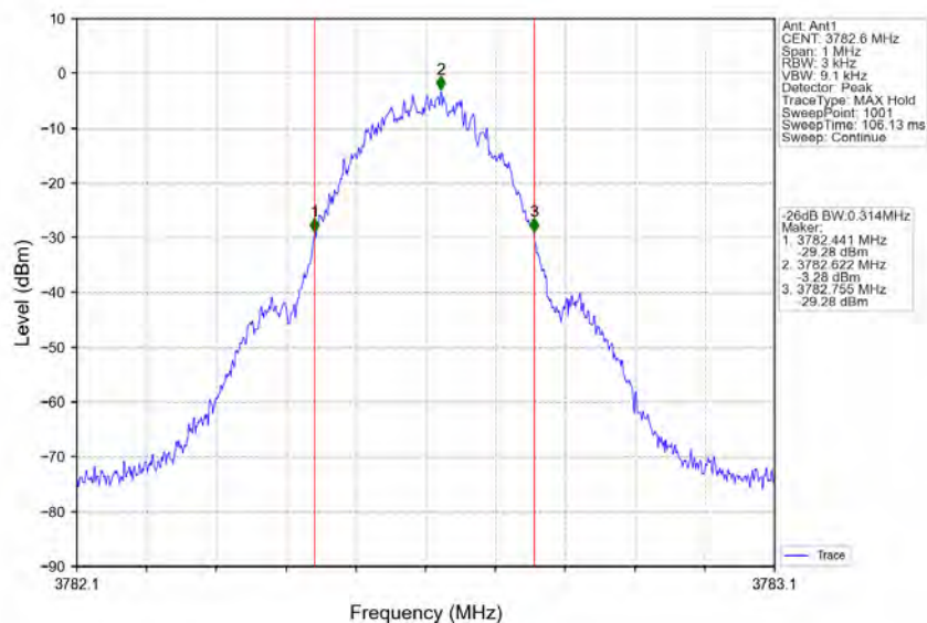
Bandn77a_3782.6MHz_GMSK_SISO_Ant1_NTNV_Input_AGC+3
