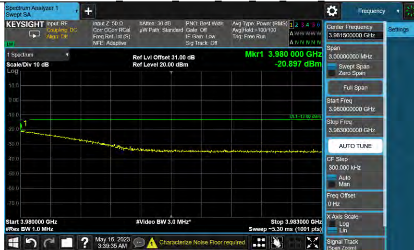
Bandn77a 3930MHz AWGN SISO Ant1 NTN AGC+3
