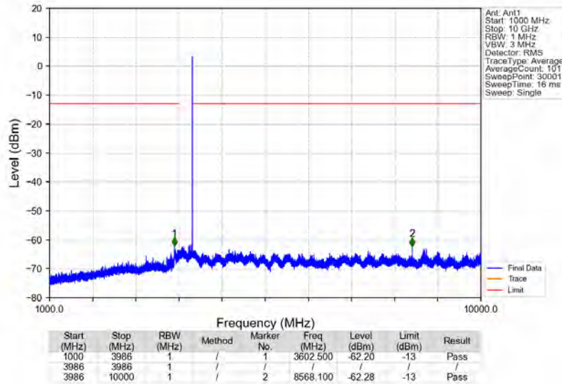
Bandn77a_3979.8MHz_GMSK_SISO_Ant1_NTNV
