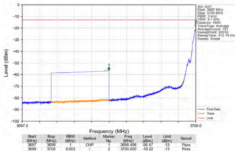
Bandn77a_3700.2MHz_GMSK_SISO_Ant1_NTNV_AGC
