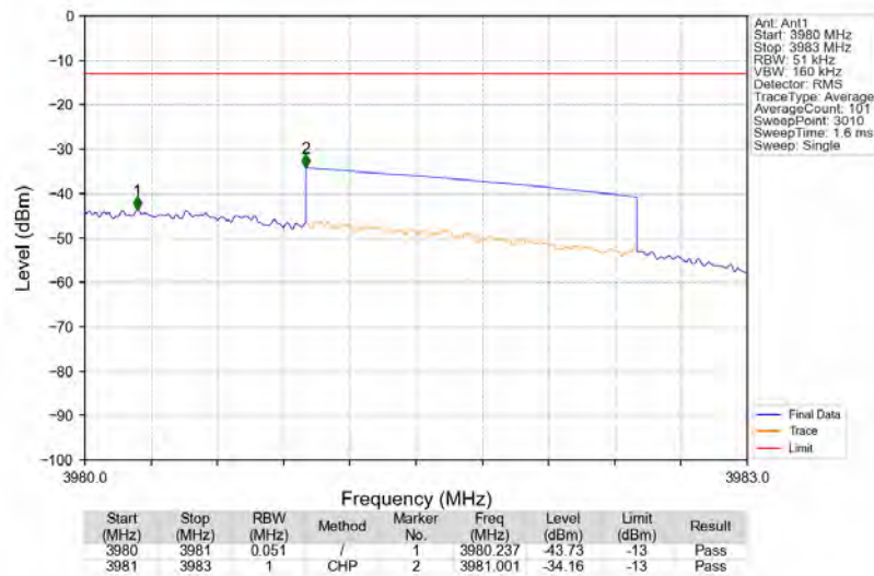
Bandn77a_3977.5MHz_AWGN_SISO_Ant1_NTNV_AGC
