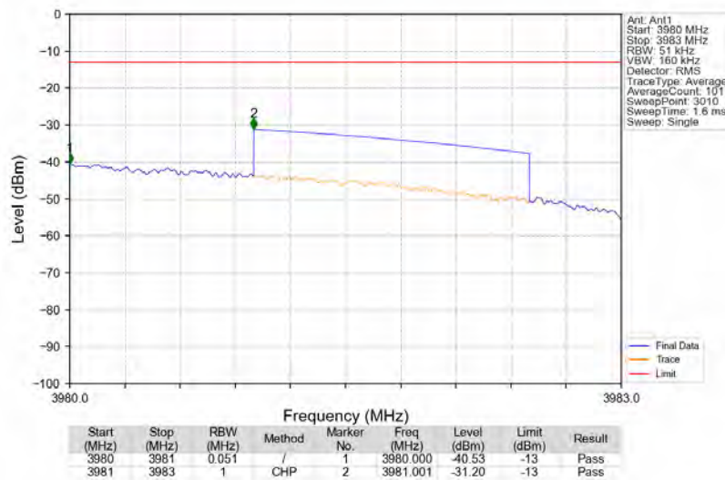
Bandn77a_3977.5MHz_AWGN_SISO_Ant1_NTNV_AGC+3
