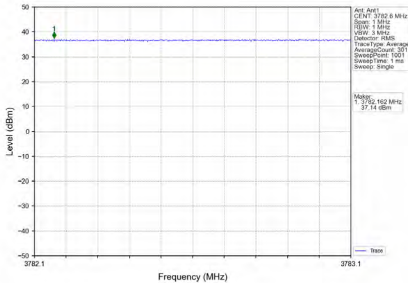
Bandn77a_3782.6MHz_GMSK_SISO_Ant1_NTNV_AGC+3
