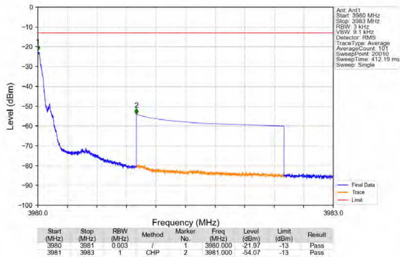
Bandn77a_3979.8MHz_GMSK_SISO_Ant1_NTNV_AGC
