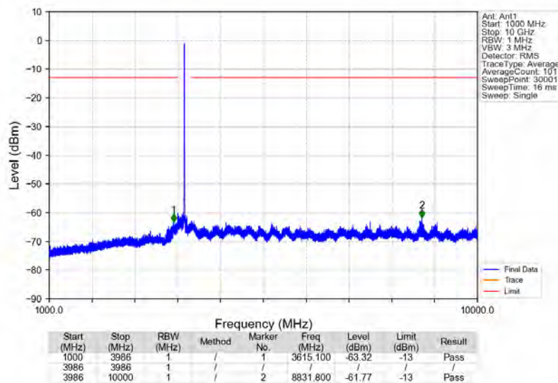
Bandn77a_3840MHz_AWGN_SISO_Ant1_NTNV
