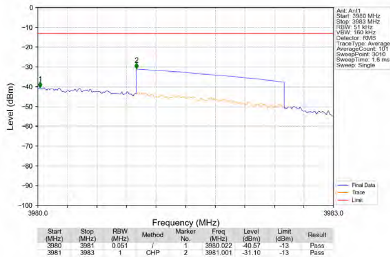
Bandn77a_3977.5MHz_AWGN_SISO_Ant1_NTNV_AGC+3
