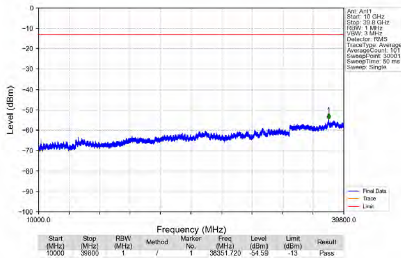
Bandn77a_3840MHz_AWGN_SISO_Ant1_NTNV
