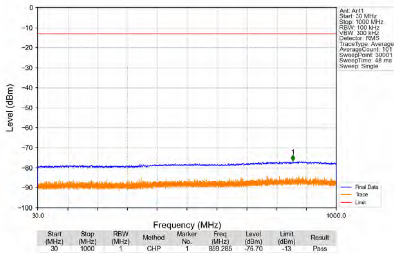
Bandn77a_3700.2MHz_GMSK_SISO_Ant1_NTNV
