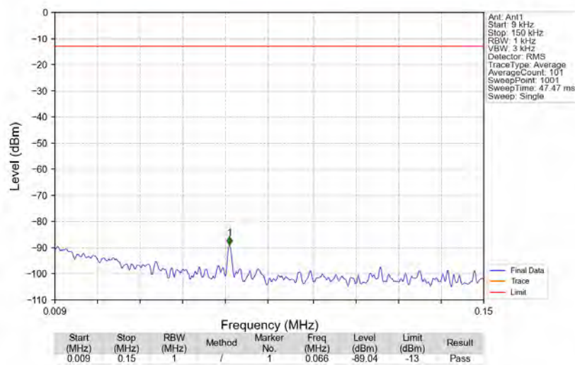
Bandn77a_3840MHz_AWGN_SISO_Ant1_NTNV
