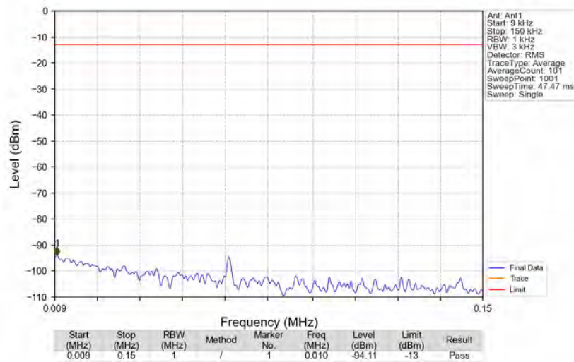
Bandn77a_3700.2MHz_GMSK_SISO_Ant1_NTNV
