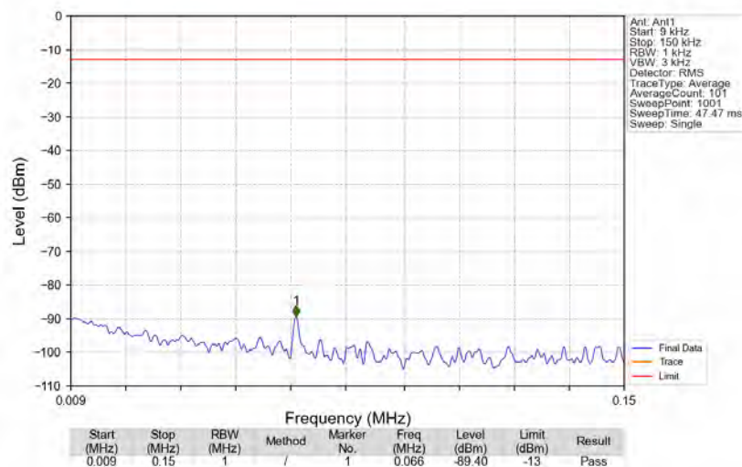
Bandn77a_3979.8MHz_GMSK_SISO_Ant1_NTNV
