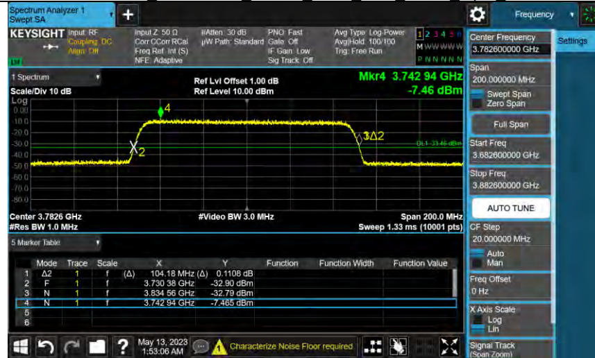
Bandn77a 3782.6MHz AWGN SISO Ant1 NTN Input AGC+
