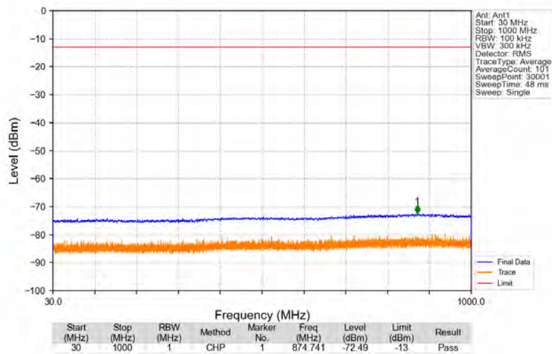
Bandn77a_3979.8MHz_GMSK_SISO_Ant1_NTNV
