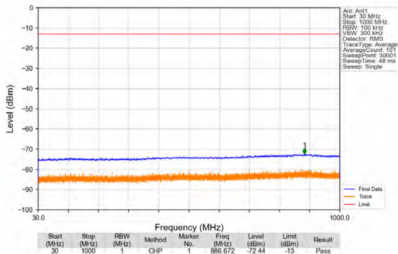
Bandn77a_3840MHz_AWGN_SISO_Ant1_NTNV
