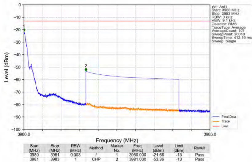
Bandn77a_3979.8MHz_GMSK_SISO_Ant1_NTNV_AGC+3
