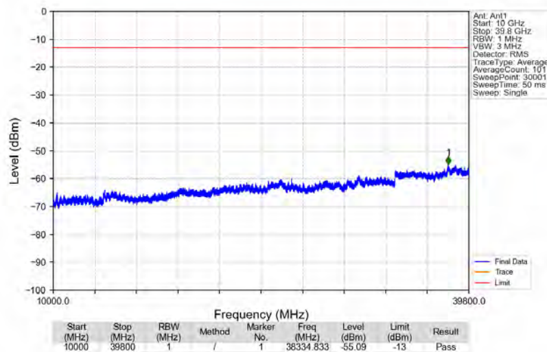
Bandn77a_3840MHz_GMSK_SISO_Ant1_NTNV
