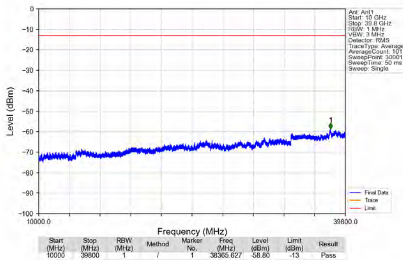
Bandn77a_3700.2MHz_GMSK_SISO_Ant1_NTNV
