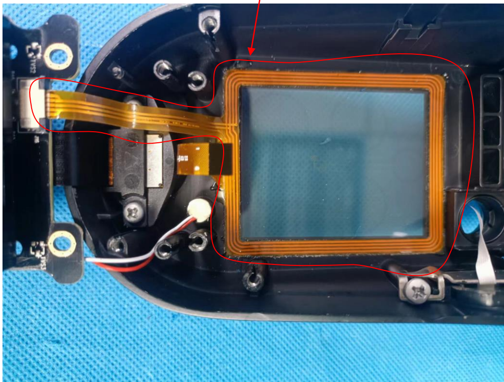
RFID antenna
