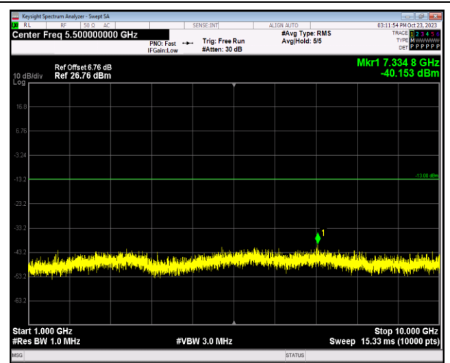
Band26-1.4MHz-QPSK-26797-1RB#0-Range2:1000~10000MHz
