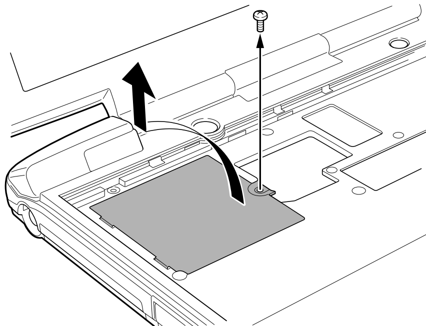
Schutzplatte entfernen
