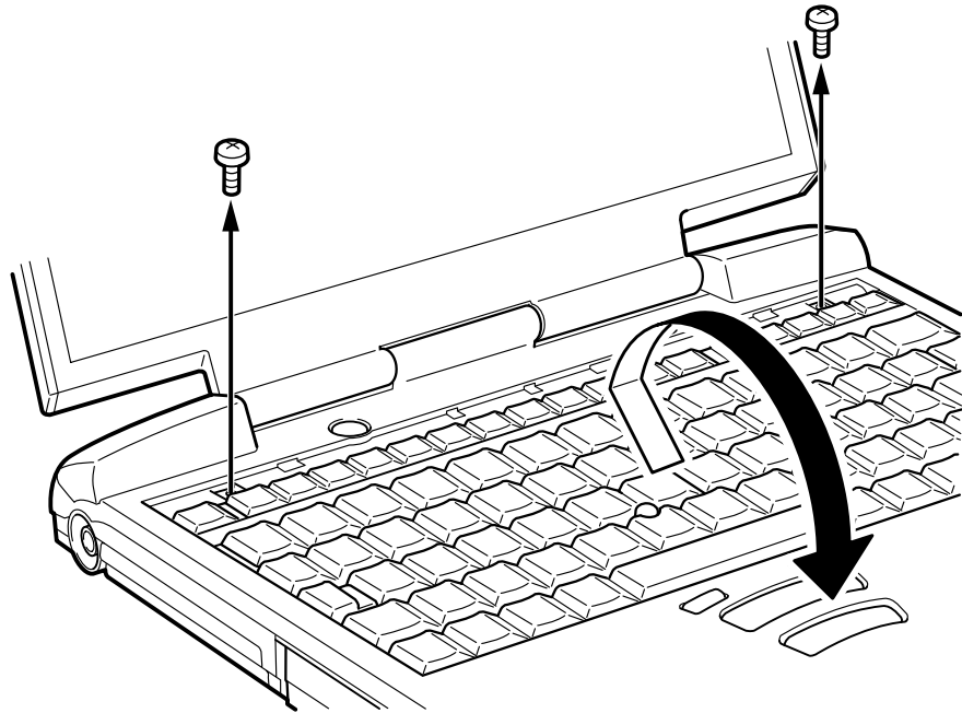
Fjerne tastaturet
