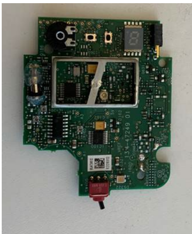
BLX1 PCB Top
