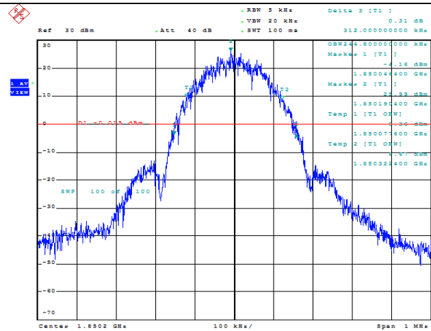
EGPRS 1900
