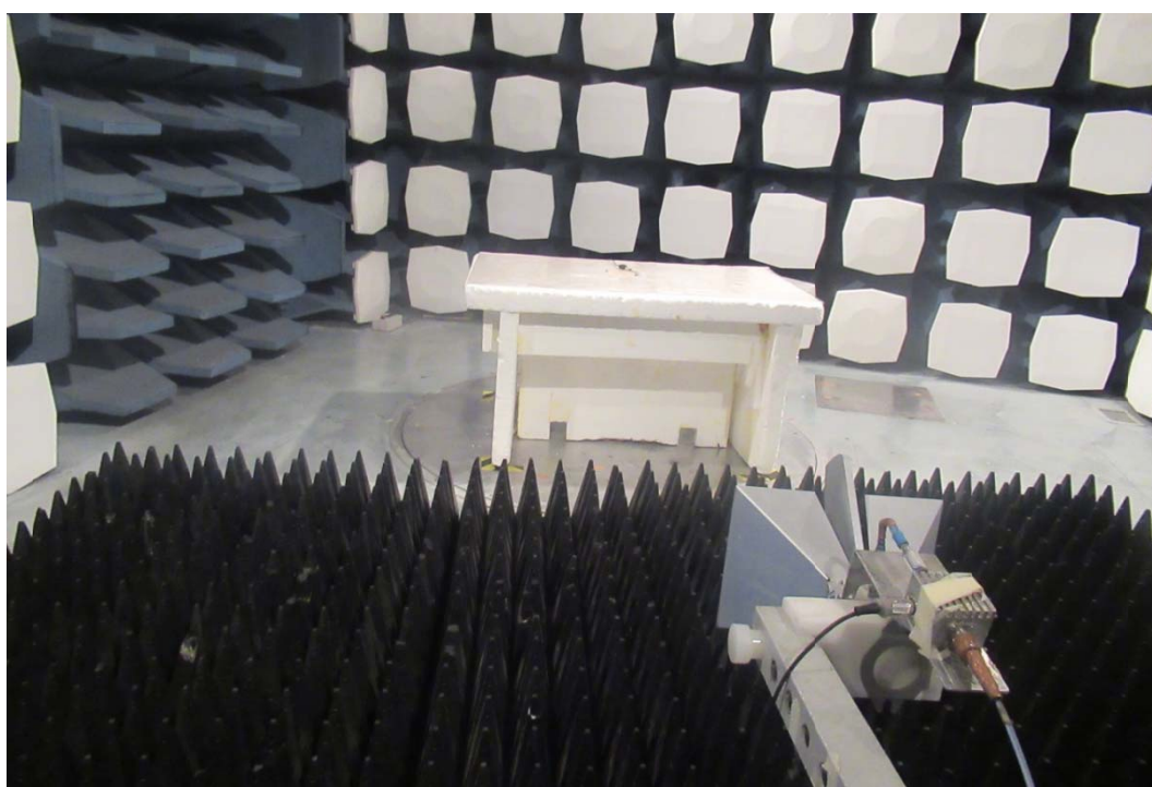
1GHz-18GHz
