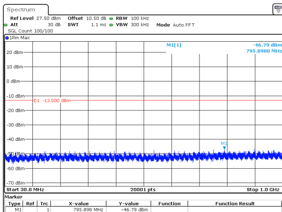
60MHz_30kHz_3770MHz_DFT-s-OFDM QPSK_RB162@0&amp;-46.79 dBm
