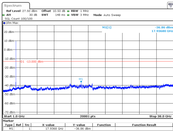
25MHz_30kHz_3787.5MHz_DFT-s-OFDM QPSK_RB1@64&amp;-36.86 dBm
