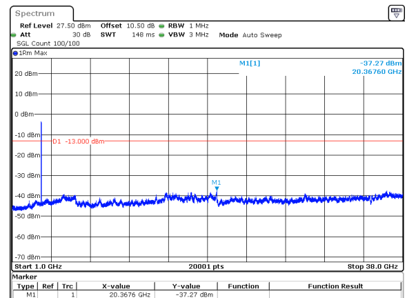
70MHz_30kHz_3735MHz_DFT-s-OFDM QPSK_RB180@0&amp;-37.27 dBm
