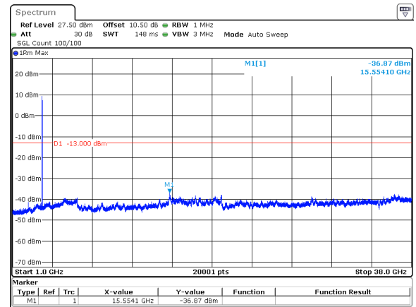
40MHz_15kHz_3720MHz_DFT-s-OFDM QPSK_RB1@215&amp;-36.87 dBm
