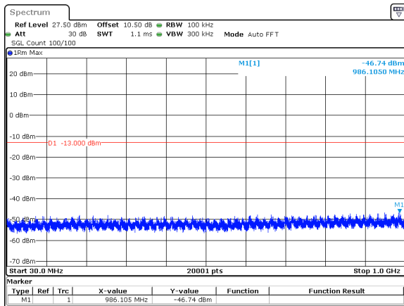
60MHz_30kHz_3770MHz_DFT-s-OFDM QPSK_RB1@161&amp;-46.74 dBm
