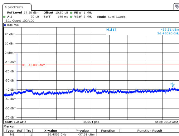
40MHz_30kHz_3780MHz_DFT-s-OFDM QPSK_RB100@0&amp;-37.31 dBm
