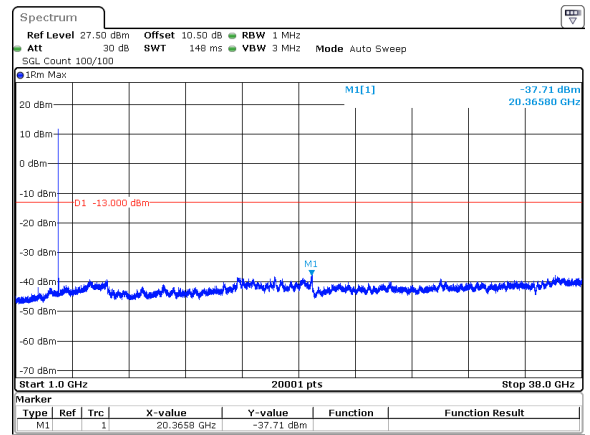
15MHz_15kHz_3792.5MHz_DFT-s-OFDM QPSK_RB1@0&amp;-37.71 dBm
