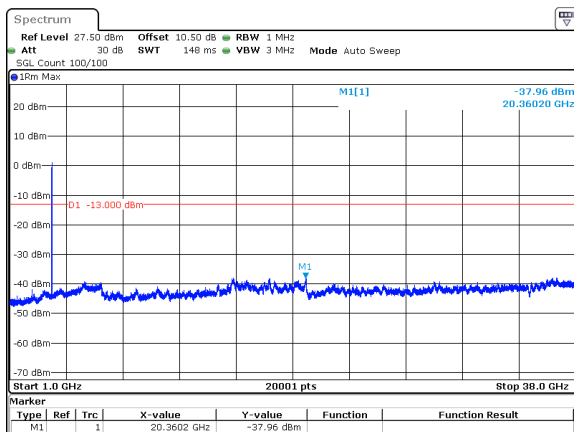
25MHz_15kHz_3750MHz_DFT-s-OFDM QPSK_RB128@0&amp;-37.96 dBm
