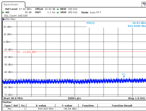
40MHz_15kHz_3720MHz_DFT-s-OFDM QPSK_RB1@215&amp;-46.84 dBm
