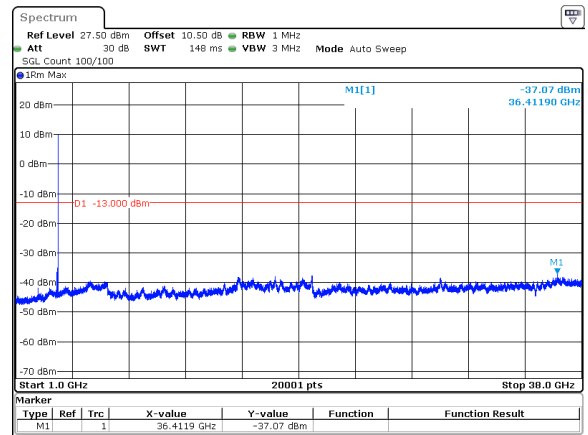
40MHz_15kHz_3750MHz_DFT-s-OFDM QPSK_RB1@215&amp;-37.07 dBm
