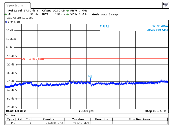
15MHz_30kHz_3707.5MHz_DFT-s-OFDM QPSK_RB1@37&amp;-37.40 dBm
