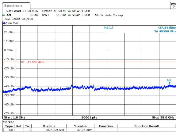
25MHz_15kHz_3712.5MHz_DFT-s-OFDM QPSK_RB128@0&amp;-37.34 dBm
