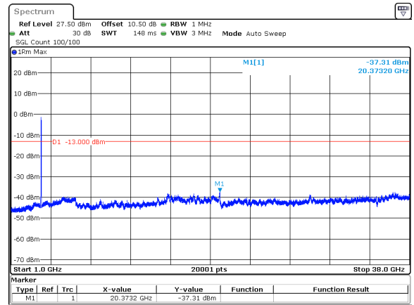
60MHz_30kHz_3770MHz_DFT-s-OFDM QPSK_RB1@0&amp;-37.31 dBm
