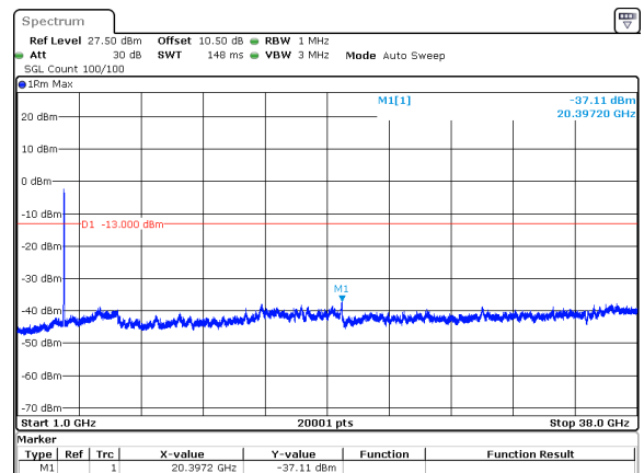
60MHz_30kHz_3770MHz_DFT-s-OFDM QPSK_RB162@0&amp;-37.11 dBm
