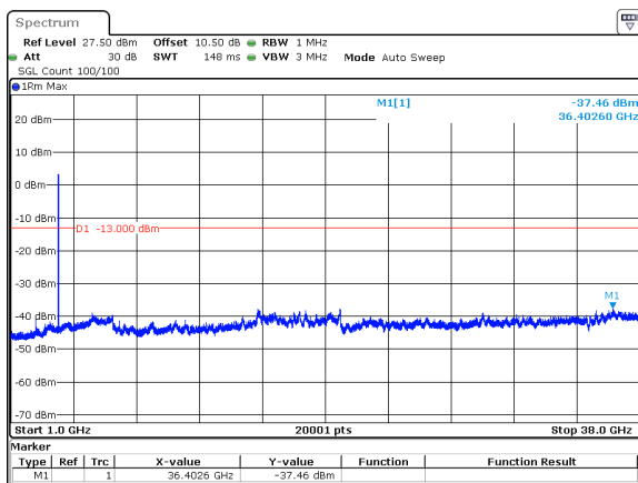
15MHz_30kHz_3792.5MHz_DFT-s-OFDM QPSK_RB36@0&amp;-37.46 dBm
