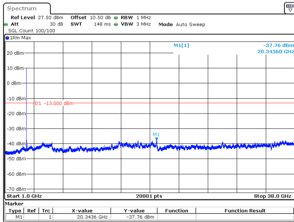
60MHz_30kHz_3750MHz_DFT-s-OFDM QPSK_RB1@0&amp;-37.76 dBm
