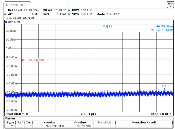
60MHz_30kHz_3750MHz_DFT-s-OFDM QPSK_RB1@0&amp;-46.73 dBm
