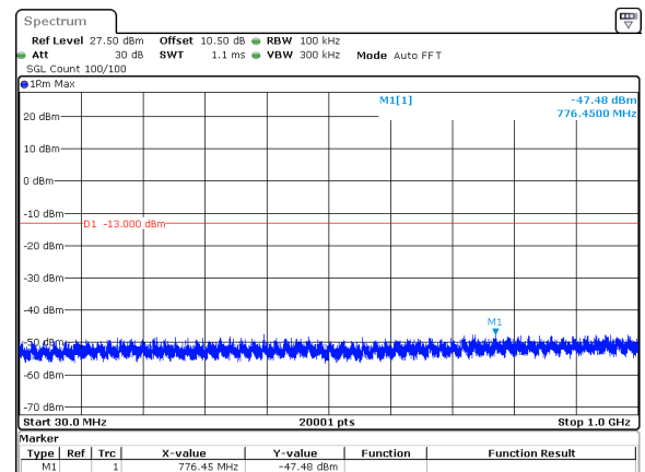
70MHz_30kHz_3750MHz_DFT-s-OFDM QPSK_RB180@0&amp;-47.48 dBm
