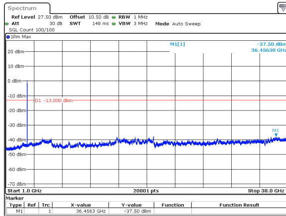
40MHz_30kHz_3780MHz_DFT-s-OFDM QPSK_RB1@0&amp;-37.50 dBm
