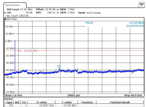
25MHz_30kHz_3787.5MHz_DFT-s-OFDM QPSK_RB64@0&amp;-37.68 dBm
