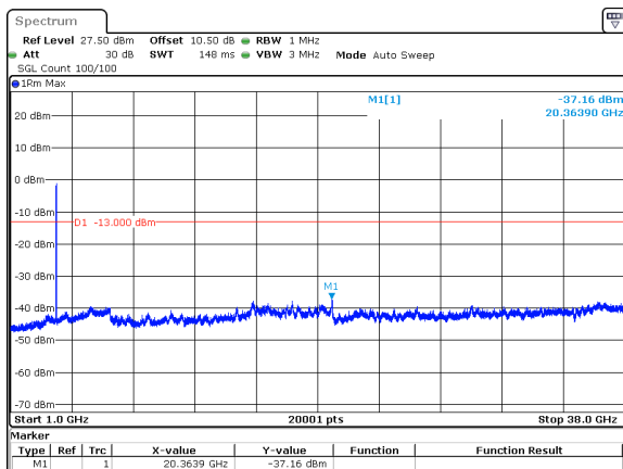
50MHz_30kHz_3725MHz_DFT-s-OFDM QPSK_RB128@0&amp;-37.16 dBm
