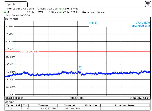
70MHz_30kHz_3765MHz_DFT-s-OFDM QPSK_RB1@0&amp;-37.49 dBm
