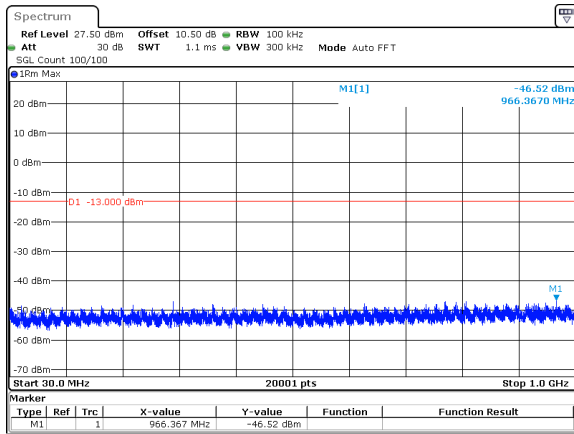
60MHz_30kHz_3770MHz_DFT-s-OFDM QPSK_RB1@0&amp;-46.52 dBm
