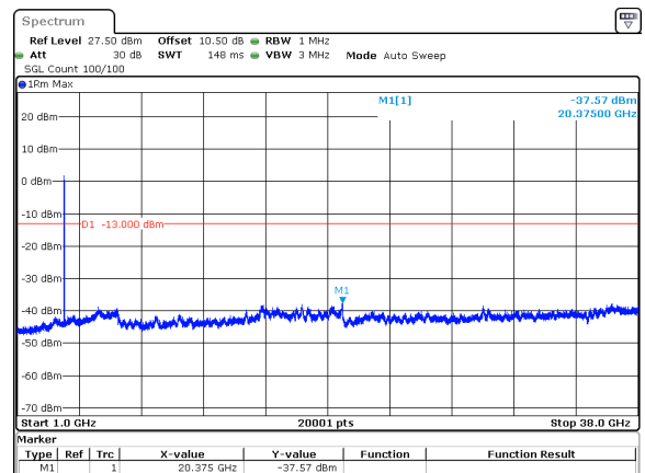
30MHz_30kHz_3785MHz_DFT-s-OFDM QPSK_RB75@0&amp;-37.57 dBm
