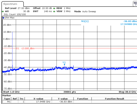
50MHz_15kHz_3725MHz_DFT-s-OFDM QPSK_RB1@0&amp;-36.83 dBm
