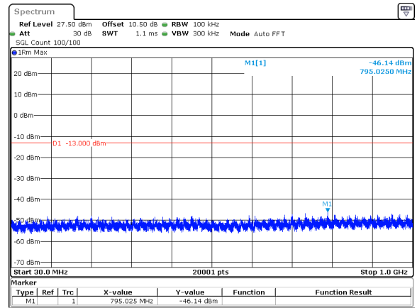
30MHz_30kHz_3785MHz_DFT-s-OFDM QPSK_RB1@0&amp;-46.14 dBm
