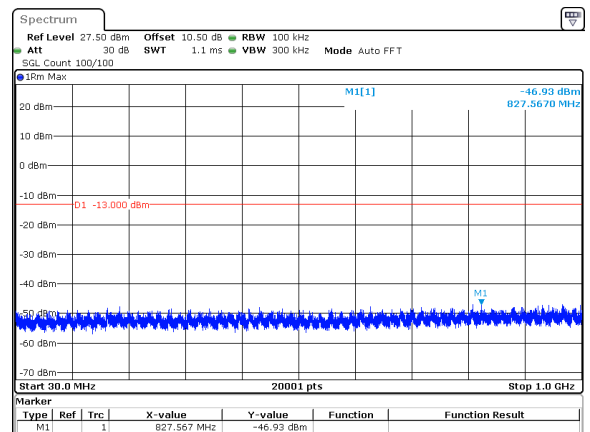
30MHz_30kHz_3750MHz_DFT-s-OFDM QPSK_RB75@0&amp;-46.93 dBm
