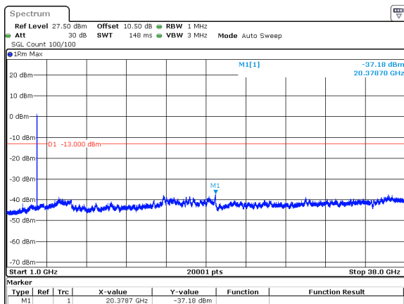
30MHz_15kHz_3785MHz_DFT-s-OFDM QPSK_RB160@0&amp;-37.18 dBm
