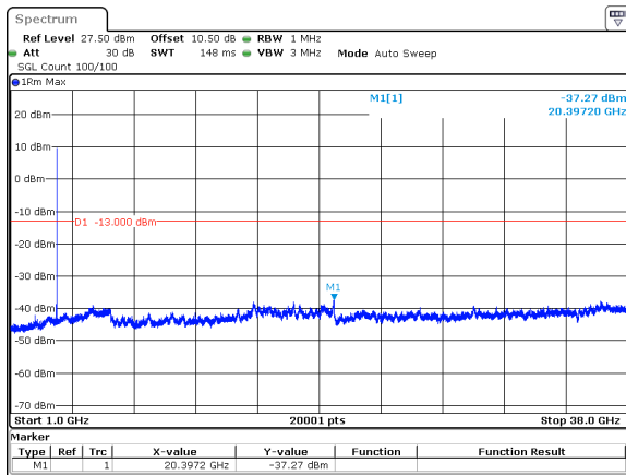
30MHz_30kHz_3750MHz_DFT-s-OFDM QPSK_RB1@77&amp;-37.27 dBm
