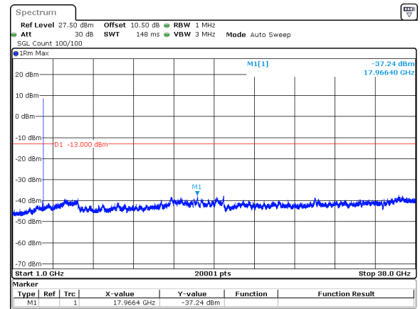
70MHz_30kHz_3765MHz_DFT-s-OFDM QPSK_RB1@188&amp;-37.24 dBm
