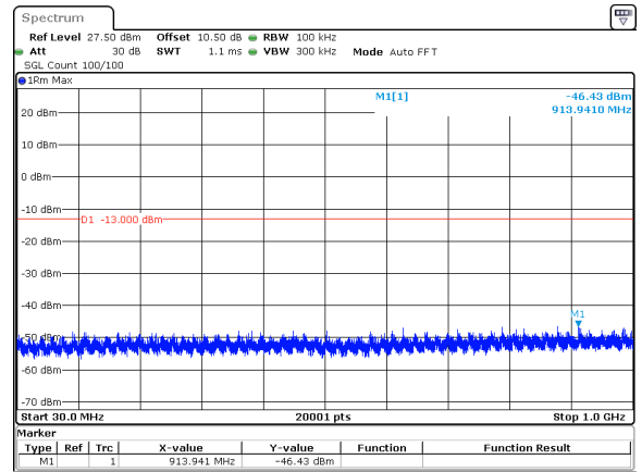
40MHz_30kHz_3720MHz_DFT-s-OFDM QPSK_RB1@0&amp;-46.43 dBm
