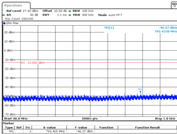
60MHz_30kHz_3750MHz_DFT-s-OFDM QPSK_RB1@161&amp;-46.37 dBm
