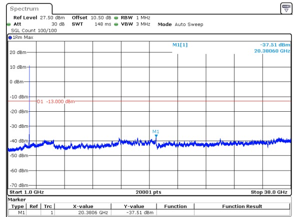
60MHz_30kHz_3770MHz_DFT-s-OFDM QPSK_RB1@161&amp;-37.51 dBm
