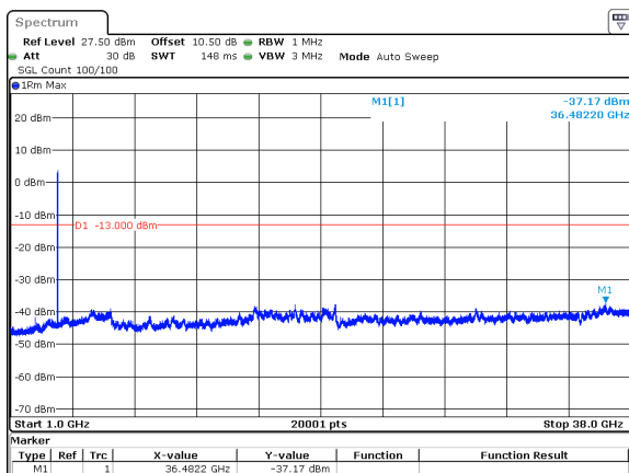
15MHz_15kHz_3792.5MHz_DFT-s-OFDM QPSK_RB75@0&amp;-37.17 dBm
