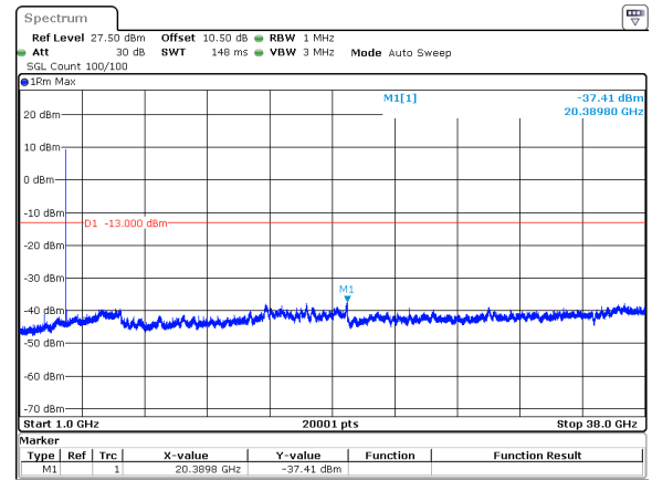
40MHz_15kHz_3720MHz_DFT-s-OFDM QPSK_RB1@0&amp;-37.41 dBm
