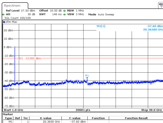
25MHz_30kHz_3750MHz_DFT-s-OFDM QPSK_RB64@0&amp;-37.60 dBm
