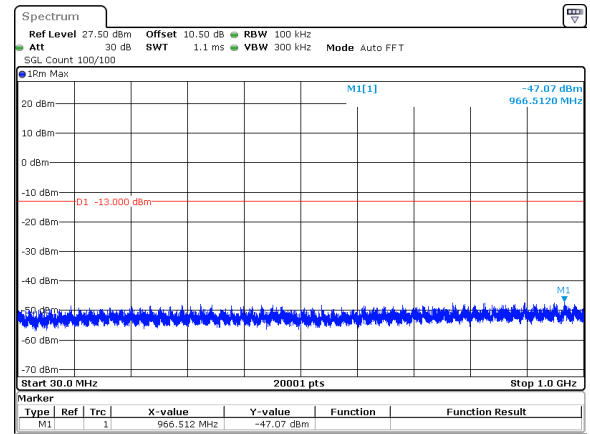
70MHz_30kHz_3750MHz_DFT-s-OFDM QPSK_RB1@0&amp;-47.07 dBm
