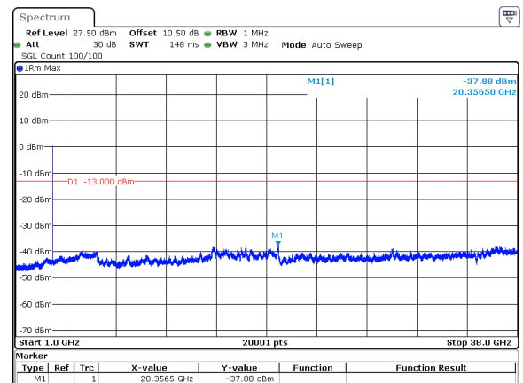
30MHz_30kHz_3715MHz_DFT-s-OFDM QPSK_RB75@0&amp;-37.88 dBm
