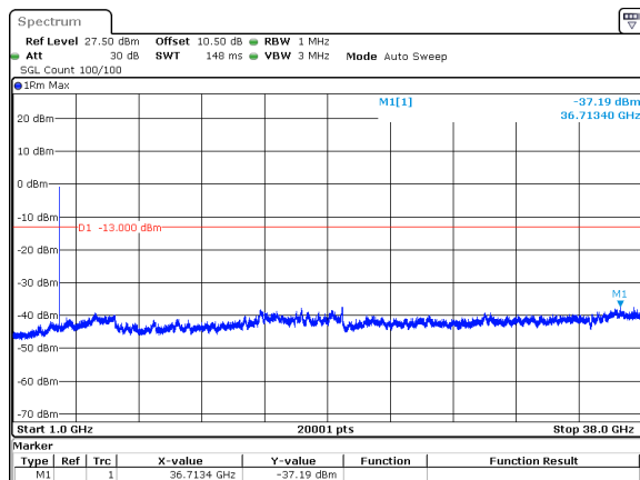
40MHz_30kHz_3720MHz_DFT-s-OFDM QPSK_RB100@0&amp;-37.19 dBm
