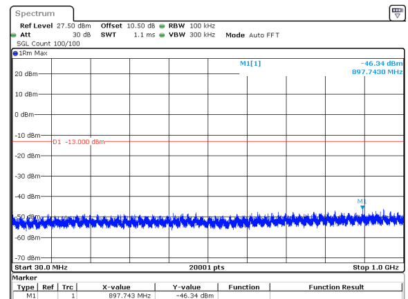
70MHz_30kHz_3765MHz_DFT-s-OFDM QPSK_RB180@0&amp;-46.34 dBm
