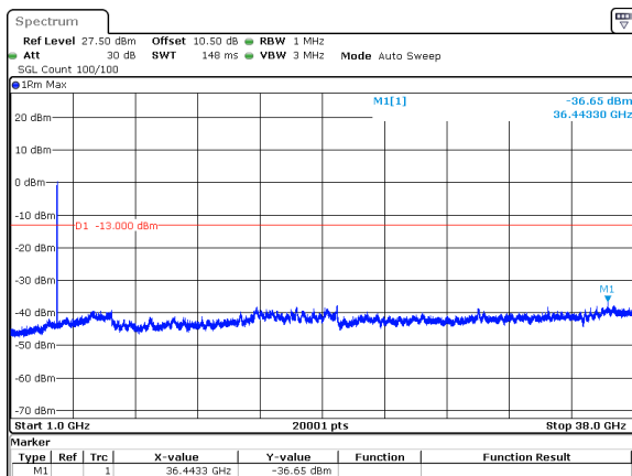
30MHz_30kHz_3750MHz_DFT-s-OFDM QPSK_RB75@0&amp;-36.65 dBm
