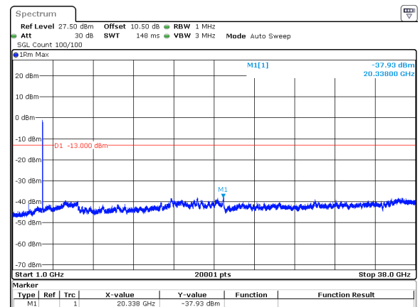
50MHz_15kHz_3725MHz_DFT-s-OFDM QPSK_RB270@0&amp;-37.93 dBm
