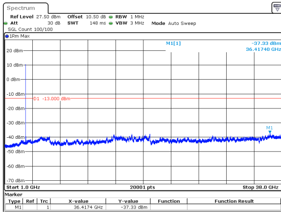
50MHz_30kHz_3775MHz_DFT-s-OFDM QPSK_RB1@0&amp;-37.33 dBm
