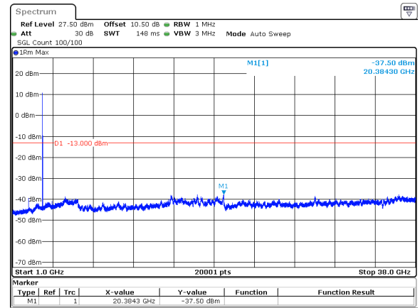
25MHz_30kHz_3750MHz_DFT-s-OFDM QPSK_RB1@0&amp;-37.50 dBm
