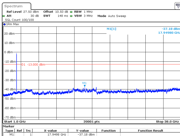
50MHz_15kHz_3775MHz_DFT-s-OFDM QPSK_RB270@0&amp;-37.18 dBm
