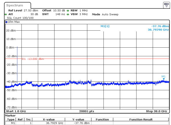
25MHz_30kHz_3712.5MHz_DFT-s-OFDM QPSK_RB64@0&amp;-37.76 dBm
