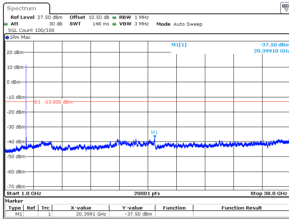
50MHz_15kHz_3750MHz_DFT-s-OFDM QPSK_RB1@0&amp;-37.50 dBm
