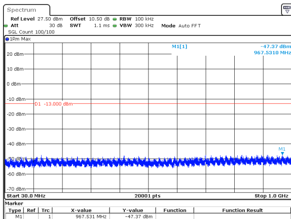
30MHz_30kHz_3785MHz_DFT-s-OFDM QPSK_RB75@0&amp;-47.37 dBm
