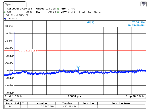
40MHz_15kHz_3780MHz_DFT-s-OFDM QPSK_RB1@0&amp;-37.58 dBm
