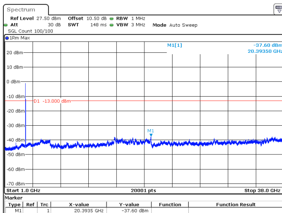
40MHz_15kHz_3720MHz_DFT-s-OFDM QPSK_RB216@0&amp;-37.60 dBm
