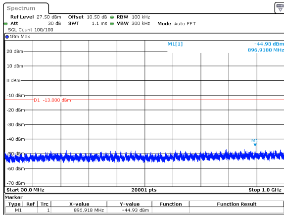
70MHz_30kHz_3765MHz_DFT-s-OFDM QPSK_RB1@0&amp;-44.93 dBm
