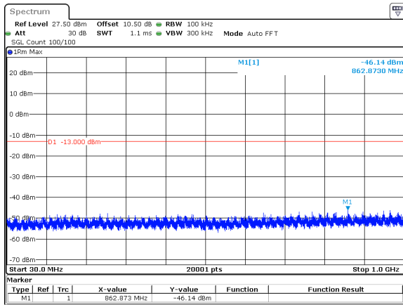
30MHz_15kHz_3785MHz_DFT-s-OFDM QPSK_RB1@0&amp;-46.14 dBm
