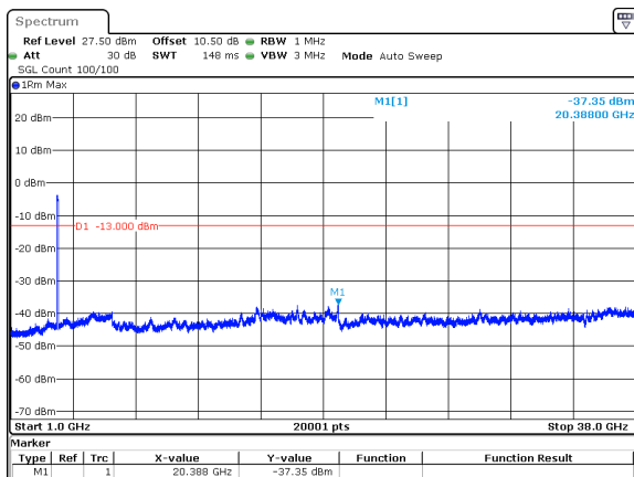
70MHz_30kHz_3765MHz_DFT-s-OFDM QPSK_RB180@0&amp;-37.35 dBm
