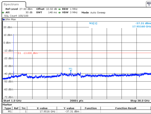
30MHz_30kHz_3750MHz_DFT-s-OFDM QPSK_RB1@0&amp;-37.31 dBm
