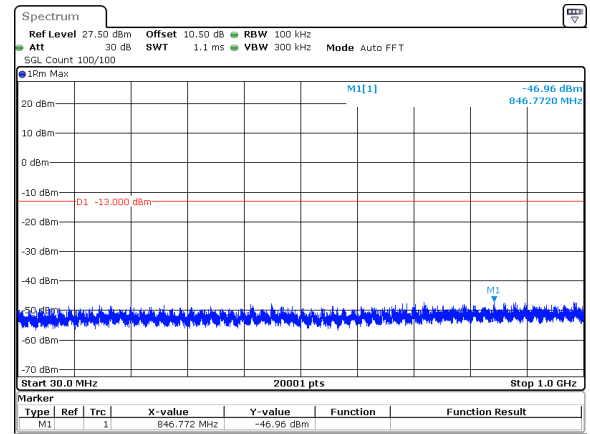
60MHz_30kHz_3730MHz_DFT-s-OFDM QPSK_RB1@0&amp;-46.96 dBm
