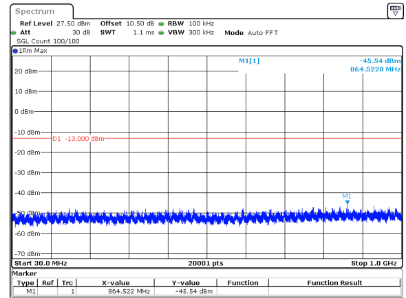
50MHz_30kHz_3750MHz_DFT-s-OFDM QPSK_RB1@0&amp;-45.54 dBm
