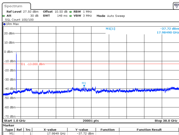
50MHz_30kHz_3775MHz_DFT-s-OFDM QPSK_RB128@0&amp;-37.72 dBm
