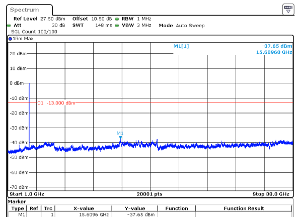
40MHz_15kHz_3750MHz_DFT-s-OFDM QPSK_RB216@0&amp;-37.65 dBm
