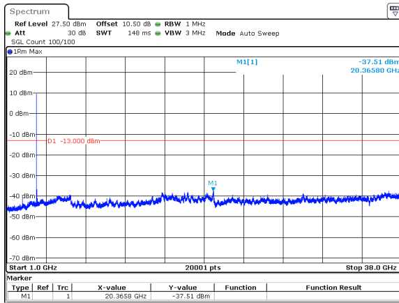
50MHz_15kHz_3775MHz_DFT-s-OFDM QPSK_RB1@0&amp;-37.51 dBm
