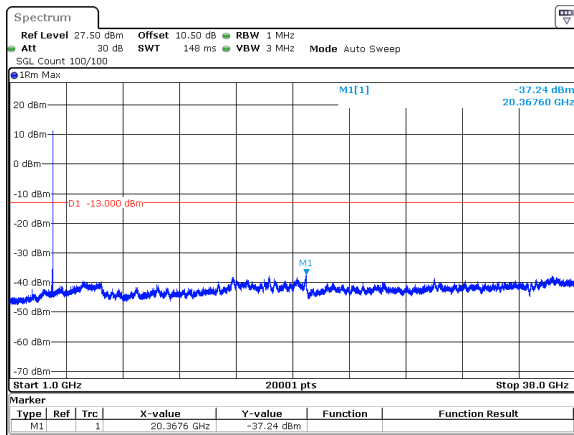
40MHz_15kHz_3780MHz_DFT-s-OFDM QPSK_RB1@215&amp;-37.24 dBm
