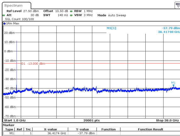
50MHz_15kHz_3775MHz_DFT-s-OFDM QPSK_RB1@269&amp;-37.79 dBm
