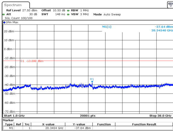
70MHz_30kHz_3750MHz_DFT-s-OFDM QPSK_RB1@0&amp;-37.64 dBm
