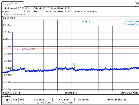
60MHz_30kHz_3730MHz_DFT-s-OFDM QPSK_RB1@0&amp;-37.05 dBm
