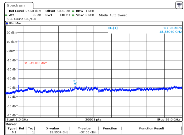
60MHz_30kHz_3730MHz_DFT-s-OFDM QPSK_RB1@161&amp;-37.06 dBm
