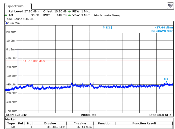
25MHz_15kHz_3787.5MHz_DFT-s-OFDM QPSK_RB128@0&amp;-37.44 dBm
