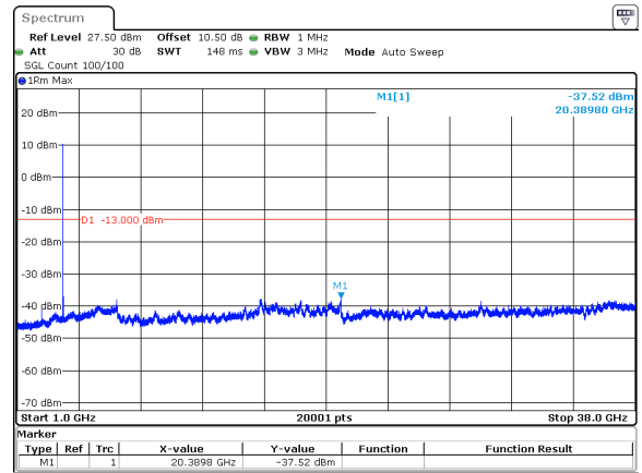
40MHz_15kHz_3750MHz_DFT-s-OFDM QPSK_RB1@0&amp;-37.52 dBm
