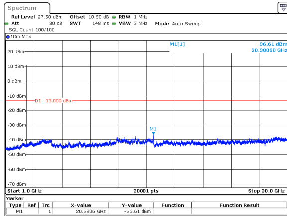
40MHz_30kHz_3720MHz_DFT-s-OFDM QPSK_RB1@0&amp;-36.61 dBm
