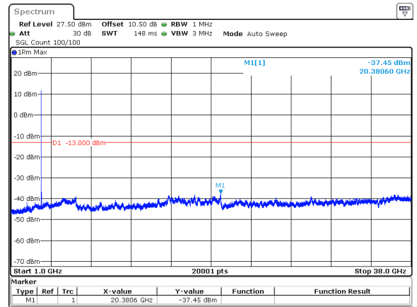
30MHz_15kHz_3785MHz_DFT-s-OFDM QPSK_RB1@0&amp;-37.45 dBm
