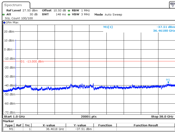
50MHz_30kHz_3750MHz_DFT-s-OFDM QPSK_RB1@0&amp;-37.51 dBm
