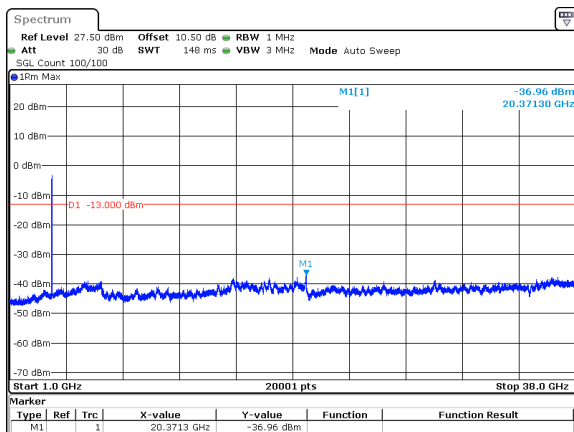
70MHz_30kHz_3750MHz_DFT-s-OFDM QPSK_RB180@0&amp;-36.96 dBm
