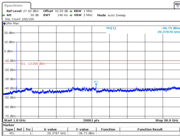
30MHz_30kHz_3785MHz_DFT-s-OFDM QPSK_RB1@77&amp;-36.73 dBm
