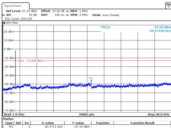
60MHz_30kHz_3750MHz_DFT-s-OFDM QPSK_RB162@0&amp;-37.33 dBm
