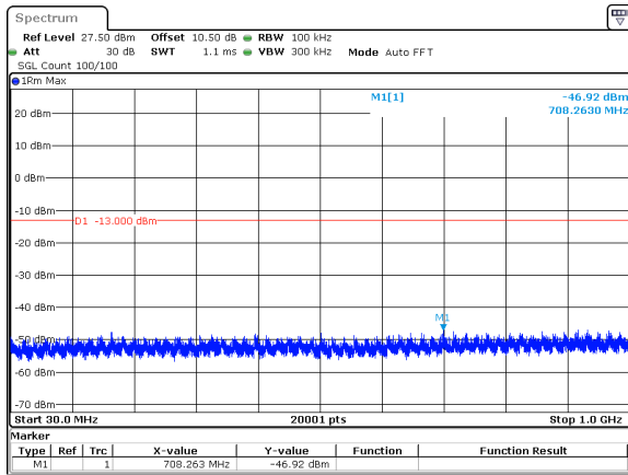
40MHz_30kHz_3750MHz_DFT-s-OFDM QPSK_RB1@0&amp;-46.92 dBm
