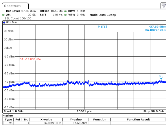
15MHz_30kHz_3707.5MHz_DFT-s-OFDM QPSK_RB36@0&amp;-37.63 dBm
