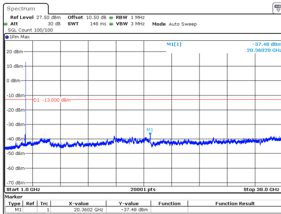
50MHz_15kHz_3750MHz_DFT-s-OFDM QPSK_RB1@269&amp;-37.48 dBm
