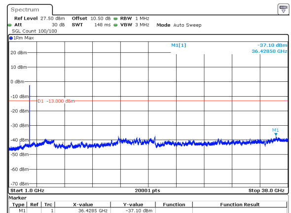
50MHz_15kHz_3750MHz_DFT-s-OFDM QPSK_RB270@0&amp;-37.10 dBm
