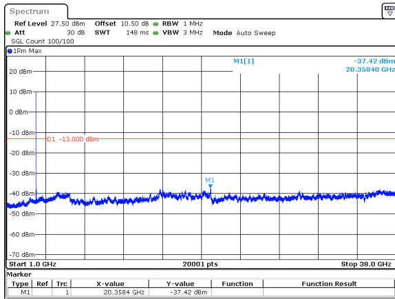
30MHz_30kHz_3785MHz_DFT-s-OFDM QPSK_RB1@0&amp;-37.42 dBm
