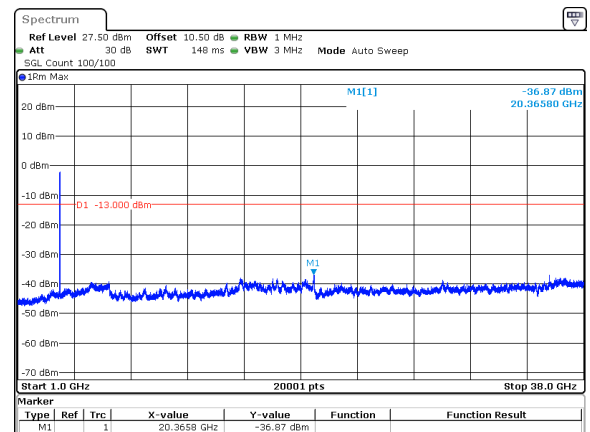
60MHz_30kHz_3730MHz_DFT-s-OFDM QPSK_RB162@0&amp;-36.87 dBm
