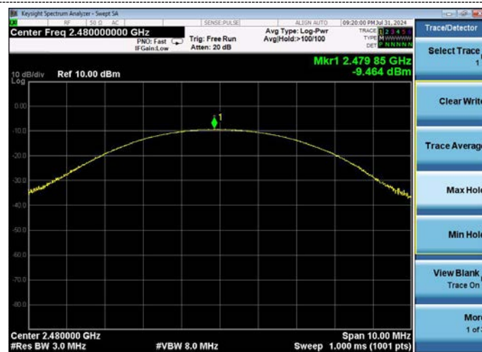
GFSK(CH78)
