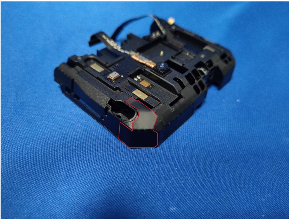
ANT 1: 5G NR TDD & LTE Diversity ANT
