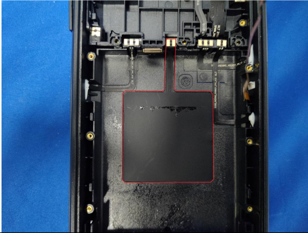
NFC ANT
