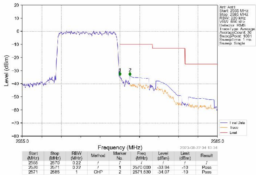
Band7 10MHz 16QAM HCH 2565MHz RB 50 0 NTV
