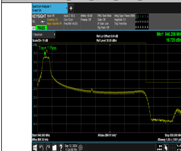
Band5_3MHz_QPSK_20635_1RB#0
