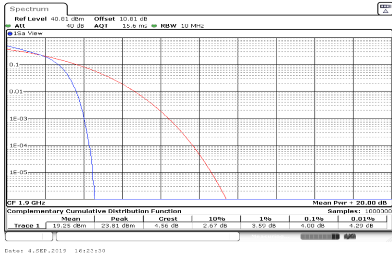
Band2-20MHz-16QAM-18700-1RB#0
