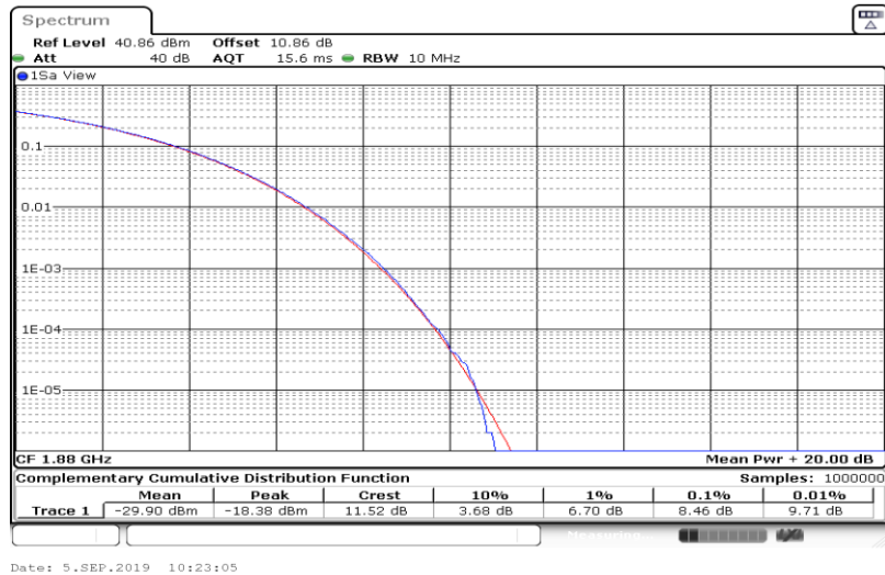
Band2-20MHz-16QAM-19100-1RB#0
