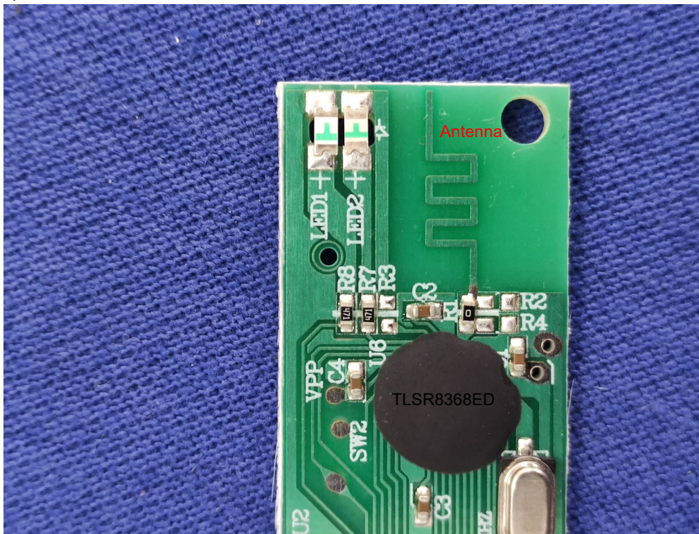
4) EUT Photo
