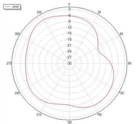
Theta=90 freq=2400MHz
