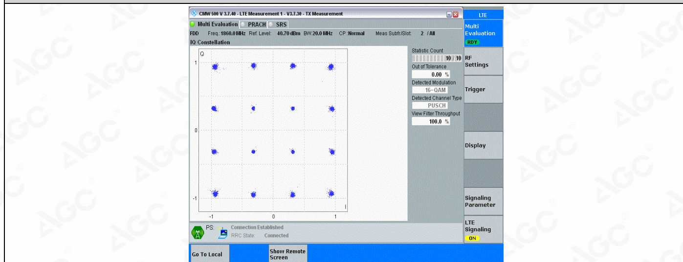
Band2-20MHz-16QAM-18900-100RB#0
