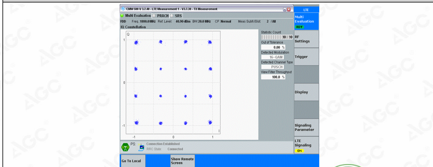
Band2-20MHz-16QAM-18900-100RB#0
