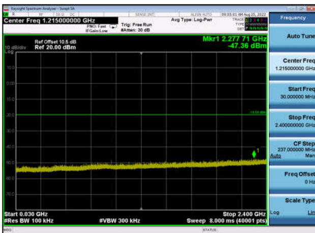
,Plot 3,30MHz~2400MHz-802.11ax(HE40) ,2452MHz,Ant0
