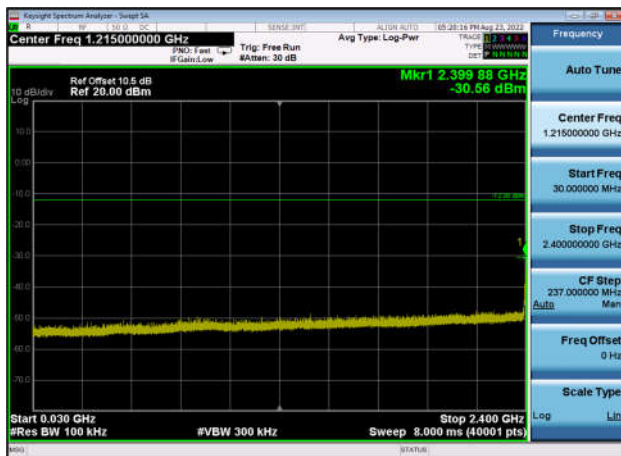
,Plot 3,30MHz~2400MHz-802.11g,2437MHz ,Ant0
