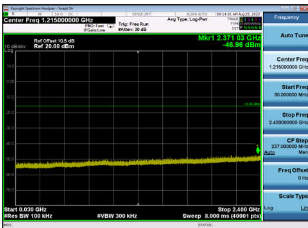
,Plot 3,30MHz~2400MHz-802.11ax(HE20) ,2462MHz,Ant0
