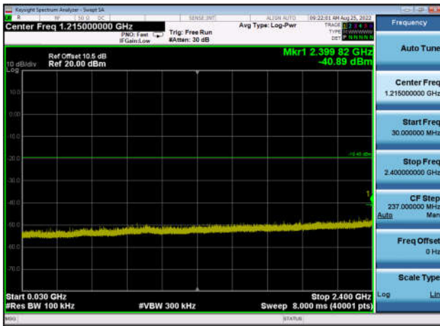
,Plot 3,30MHz~2400MHz-802.11ax(HE40) ,2437MHz,Ant0
