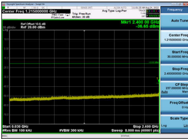
,Plot 3,30MHz~2400MHz-802.11ax(HE20) ,2437MHz,Ant0
