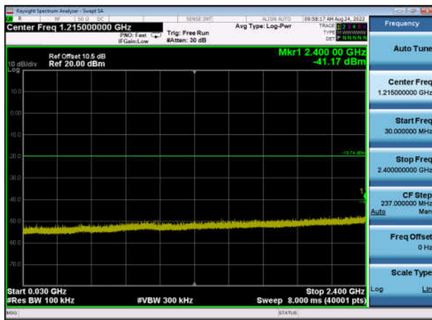
,Plot 3,30MHz~2400MHz-802.11n(HT40) ,2437MHz,Ant0
