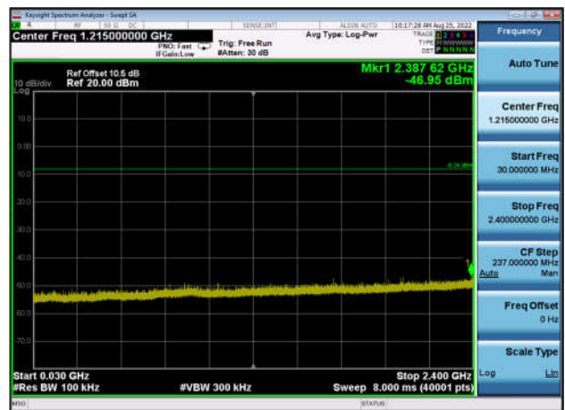
,Plot 3,30MHz~2400MHz-802.11b,2462MHz ,Ant1
