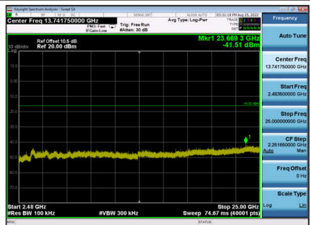
,Plot 4,2483.5MHz~25000MHz-802.11ax(H T20),2462MHz,Ant1
