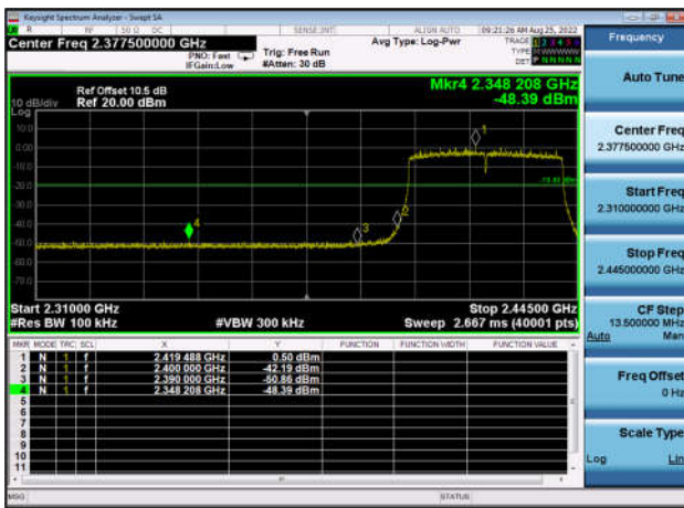
,Plot 2,Band Edge-802.11ax(HE40) ,2437MHz,Ant0
