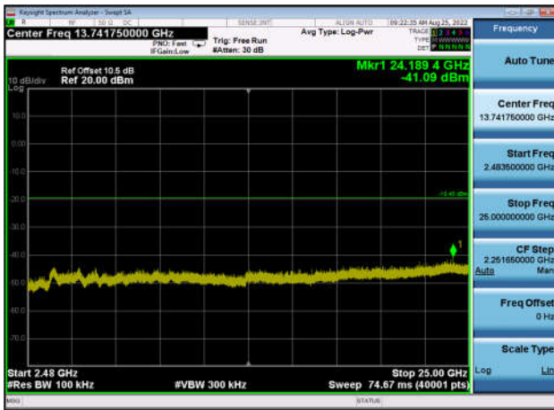
,Plot 4,2483.5MHz~25000MHz-802.11ax(H T40),2437MHz,Ant0
