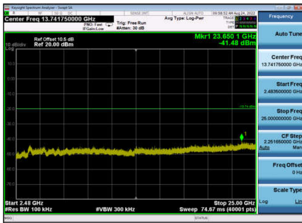
,Plot 4,2483.5MHz~25000MHz-802.11n(HT 40),2437MHz,Ant0
