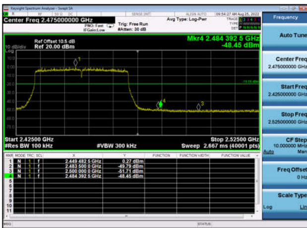
,Plot 2,Band Edge-802.11ax(HE40) ,2452MHz,Ant0
