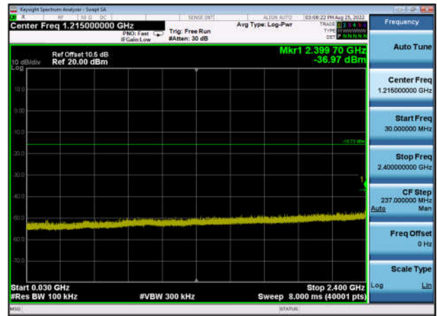
,Plot 3,30MHz~2400MHz-802.11ax(HE20) ,2437MHz,Ant1
