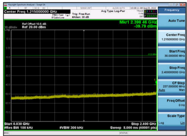
,Plot 3,30MHz~2400MHz-802.11b,2437MHz ,Ant1
