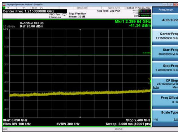
,Plot 3,30MHz~2400MHz-802.11b,2437MHz ,Ant0
