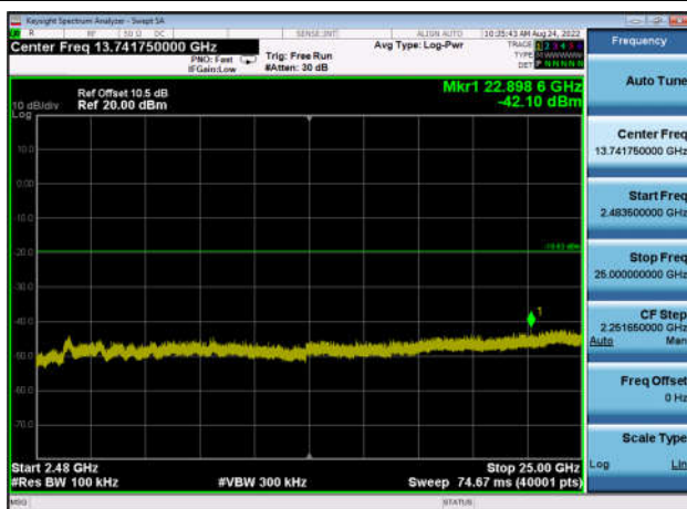
,Plot 4,2483.5MHz~25000MHz-802.11n(HT 40),2452MHz,Ant0
