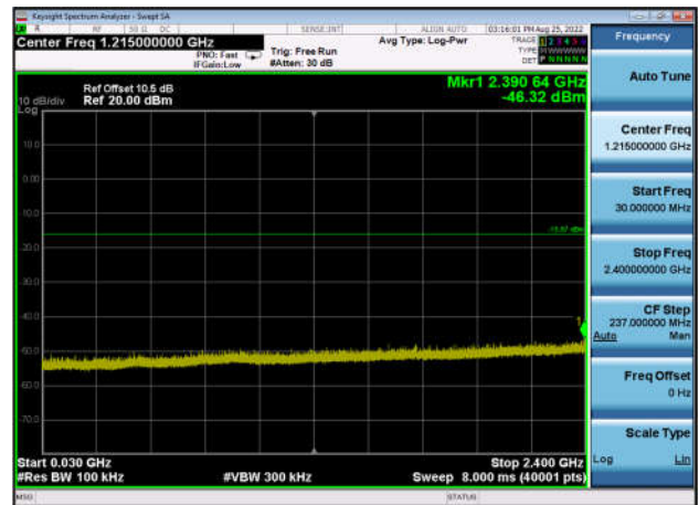
,Plot 3,30MHz~2400MHz-802.11ax(HE20) ,2462MHz,Ant1
