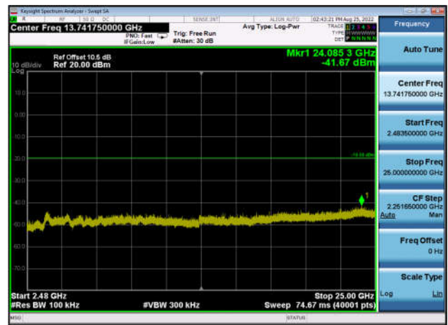
,Plot 4,2483.5MHz~25000MHz-802.11n(HT 40),2437MHz,Ant1
