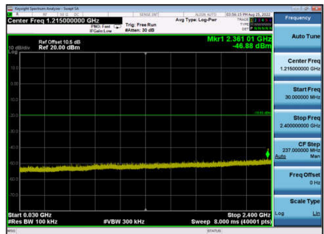
,Plot 3,30MHz~2400MHz-802.11ax(HE40) ,2452MHz,Ant1
