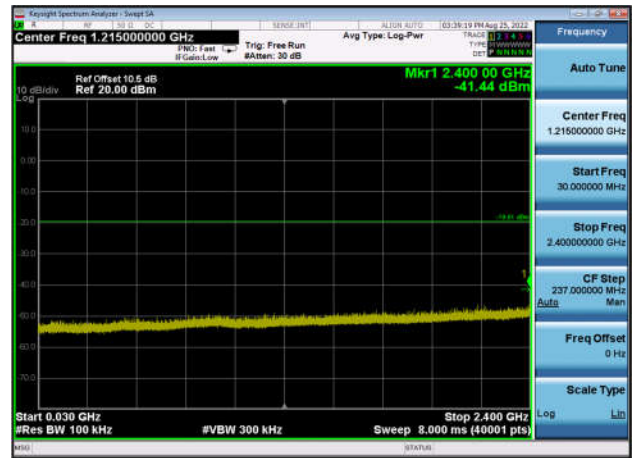
,Plot 3,30MHz~2400MHz-802.11ax(HE40) ,2437MHz,Ant1
