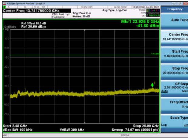
,Plot 4,2483.5MHz~25000MHz-802.11b ,2462MHz,Ant0
