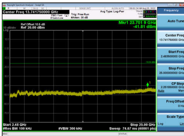
,Plot 4,2483.5MHz~25000MHz-802.11ax(H T20),2462MHz,Ant0
