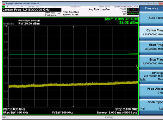
,Plot 3,30MHz~2400MHz-802.11n(HT20) ,2437MHz,Ant0
