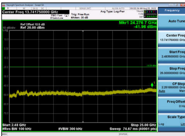
,Plot 4,2483.5MHz~25000MHz-802.11ax(H T40),2452MHz,Ant0
