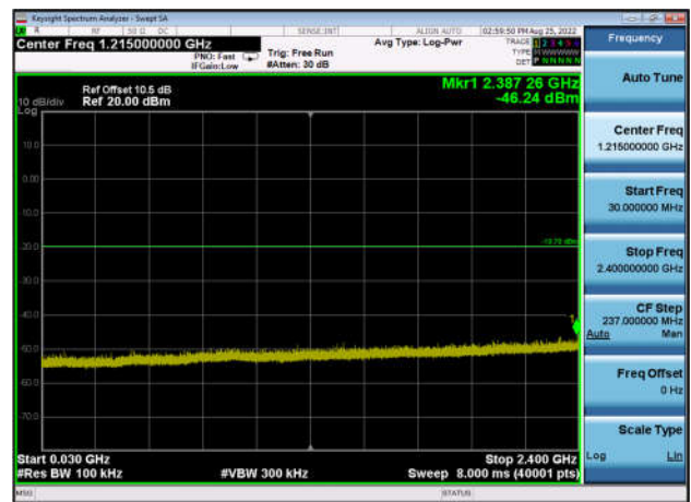
,Plot 3,30MHz~2400MHz-802.11n(HT40) ,2452MHz,Ant1
