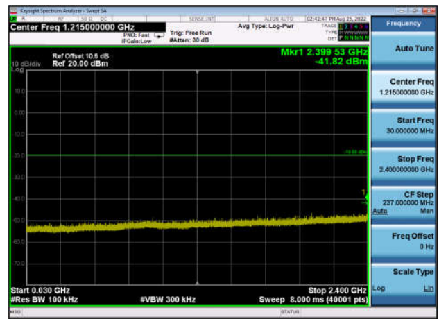
,Plot 3,30MHz~2400MHz-802.11n(HT40) ,2437MHz,Ant1
