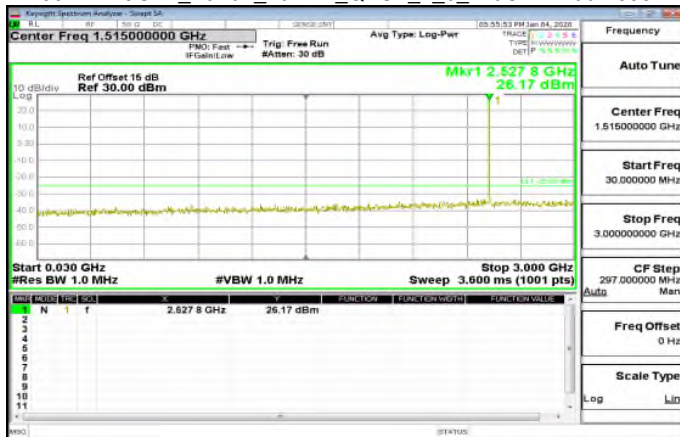
30MHz~3GHz_Band7_20MHz_QPSK_1_0_MidCH21100-2535
