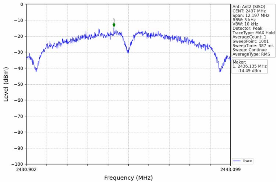
802.11b_MCH_2437MHz_Ant2 (SISO)_NTNV
