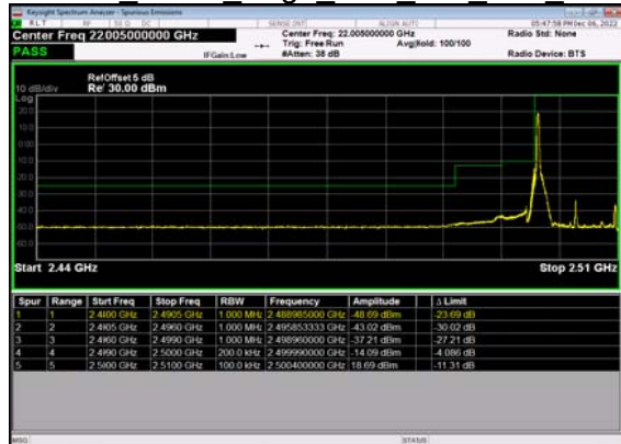
N7(10M)_DFT-s-OFDM BPSK Edge 1RB Left Low CH
