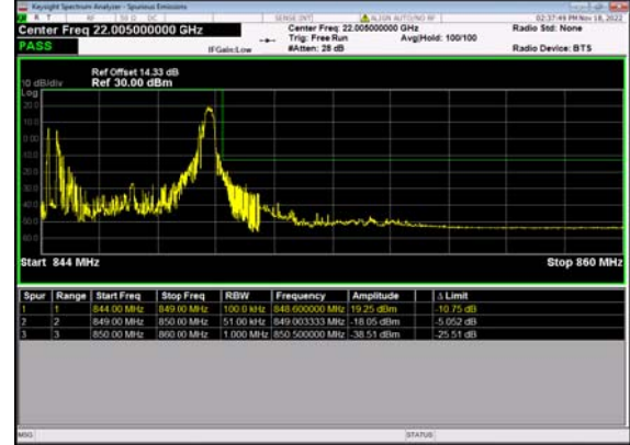
N5(5M)_DFT-s- OFDM QPSK Edge 1RB Right High CH
