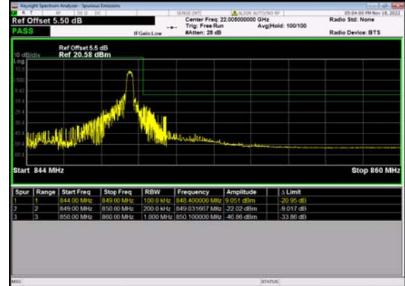
N5(20M)_DFT-s-OFDM QPSK Edge 1RB Right High CH
