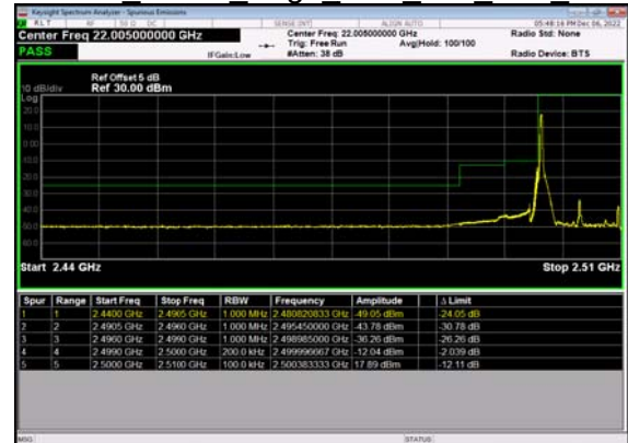
N7(10M)_DFT-s-OFDM QPSK Edge 1RB Left Low CH
